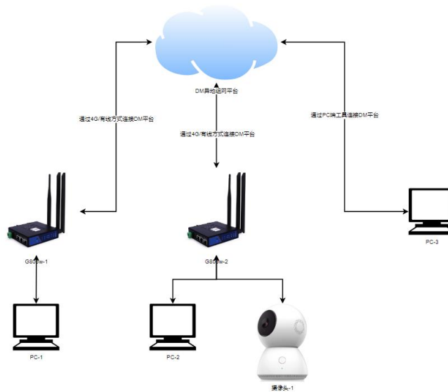
图 6 组网拓扑
