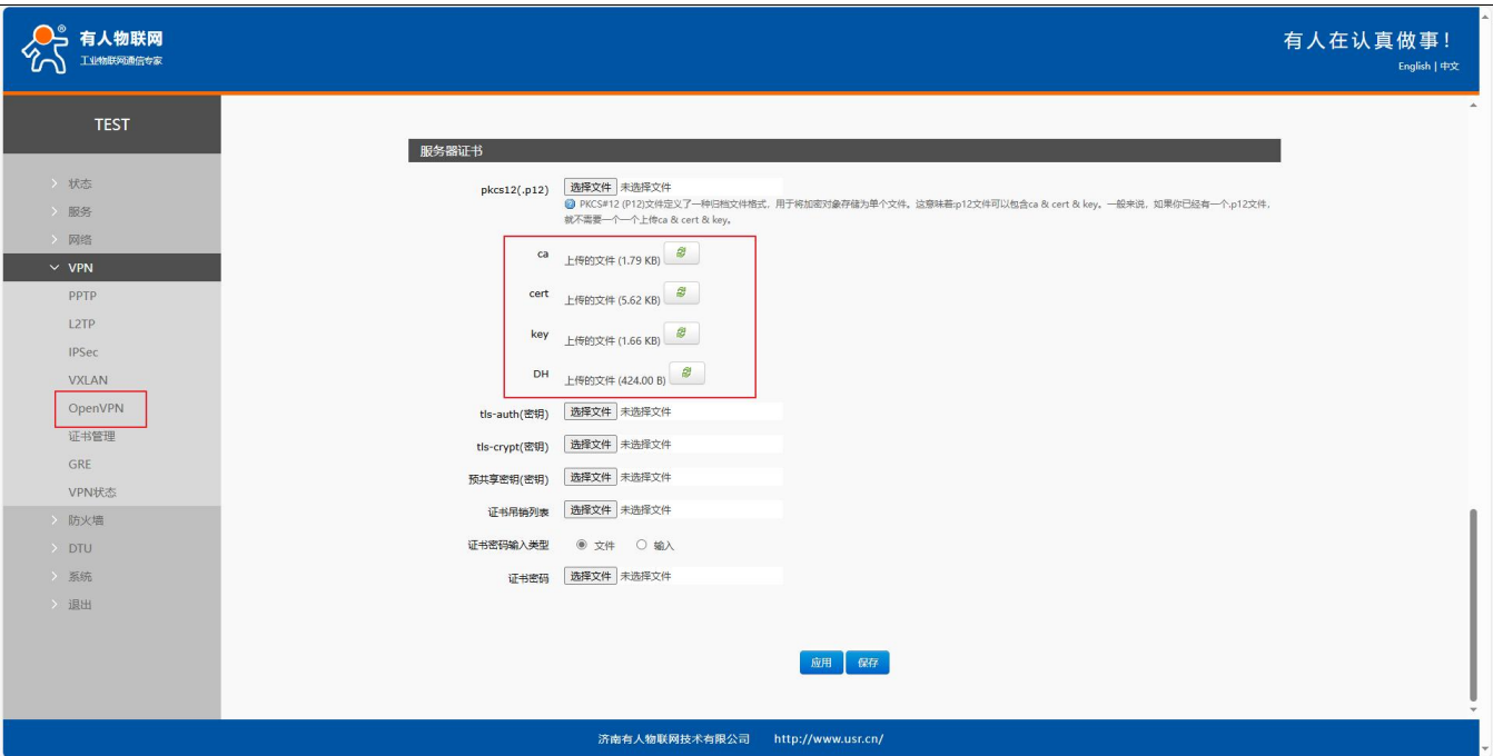
图 54 Openvpn 配置 3
