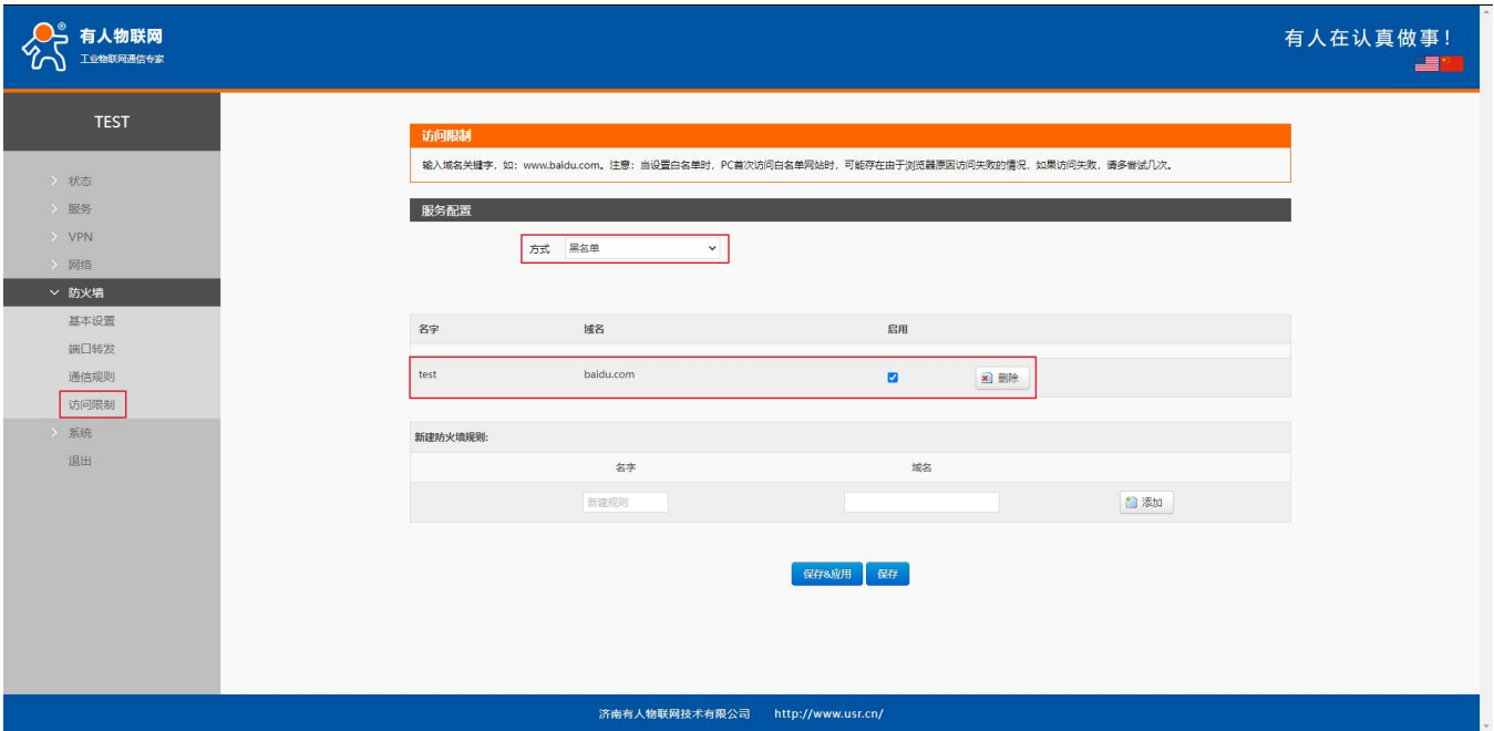
图 89 域名黑名单
