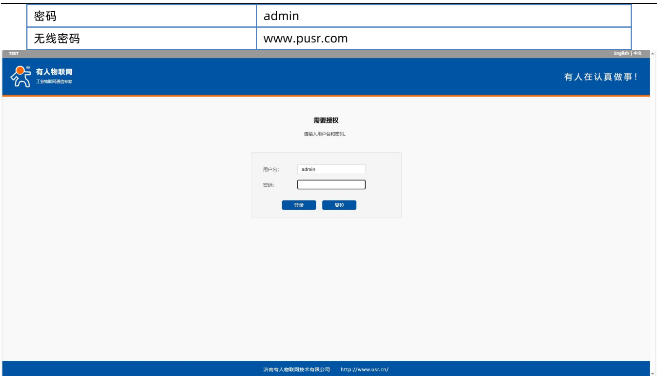
图 3 登录首页
