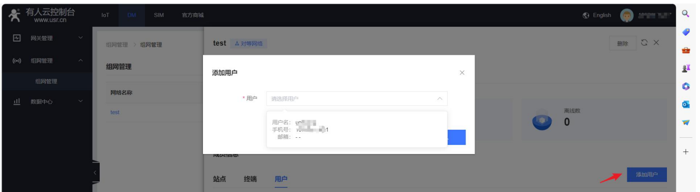
图 12 添加用户
