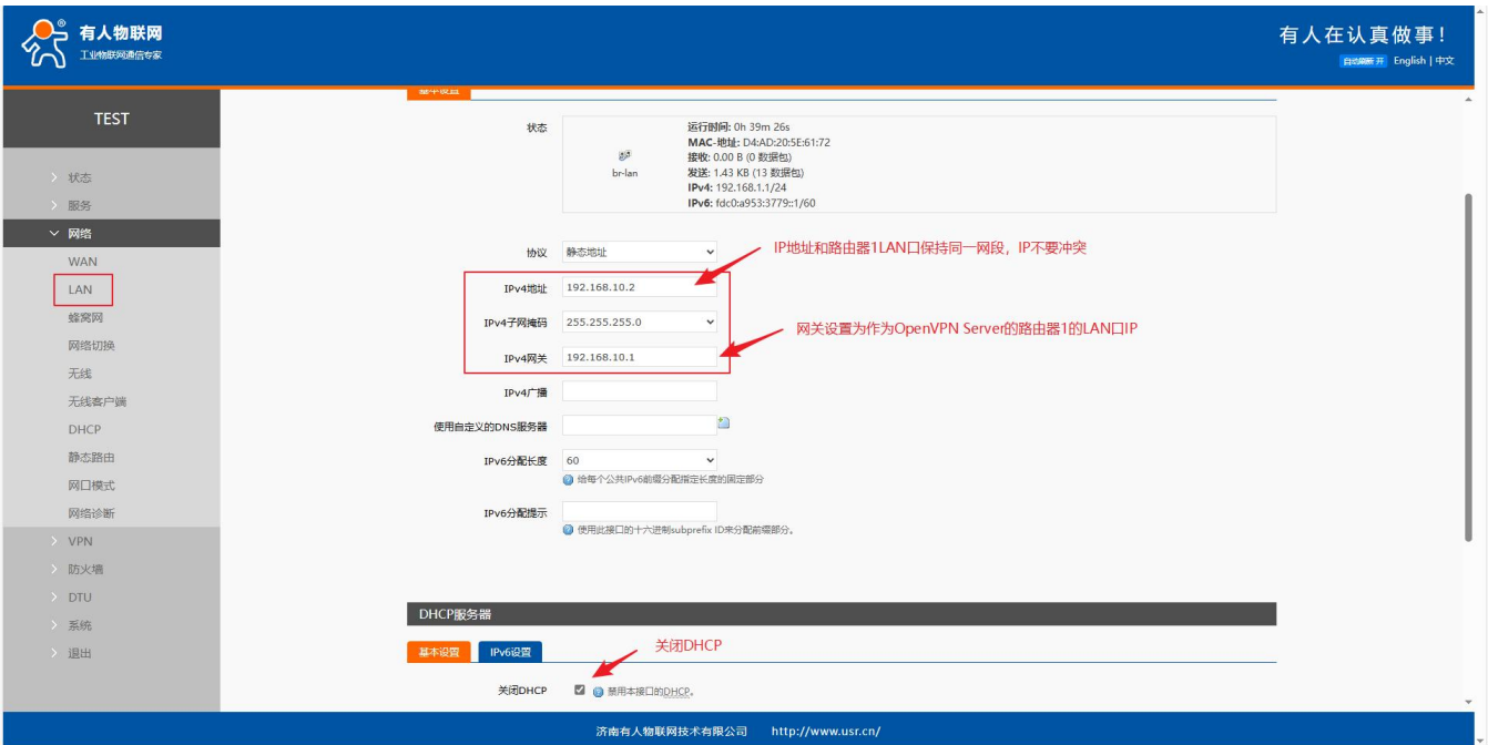
图 55 LAN 口配置
