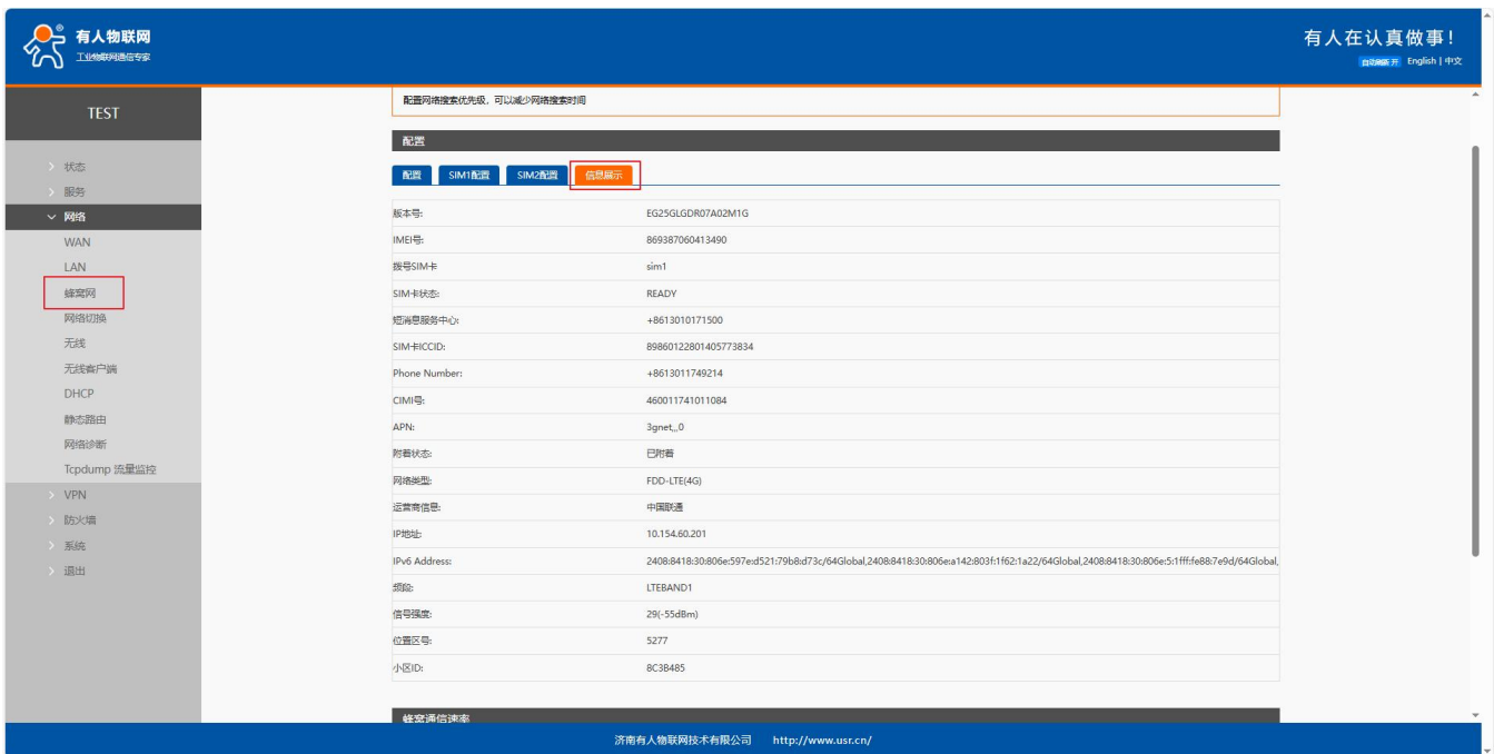
图 23 SIM 显示
