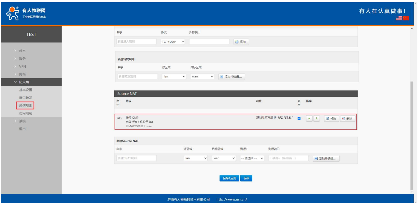
图 83 NAT 设置三
