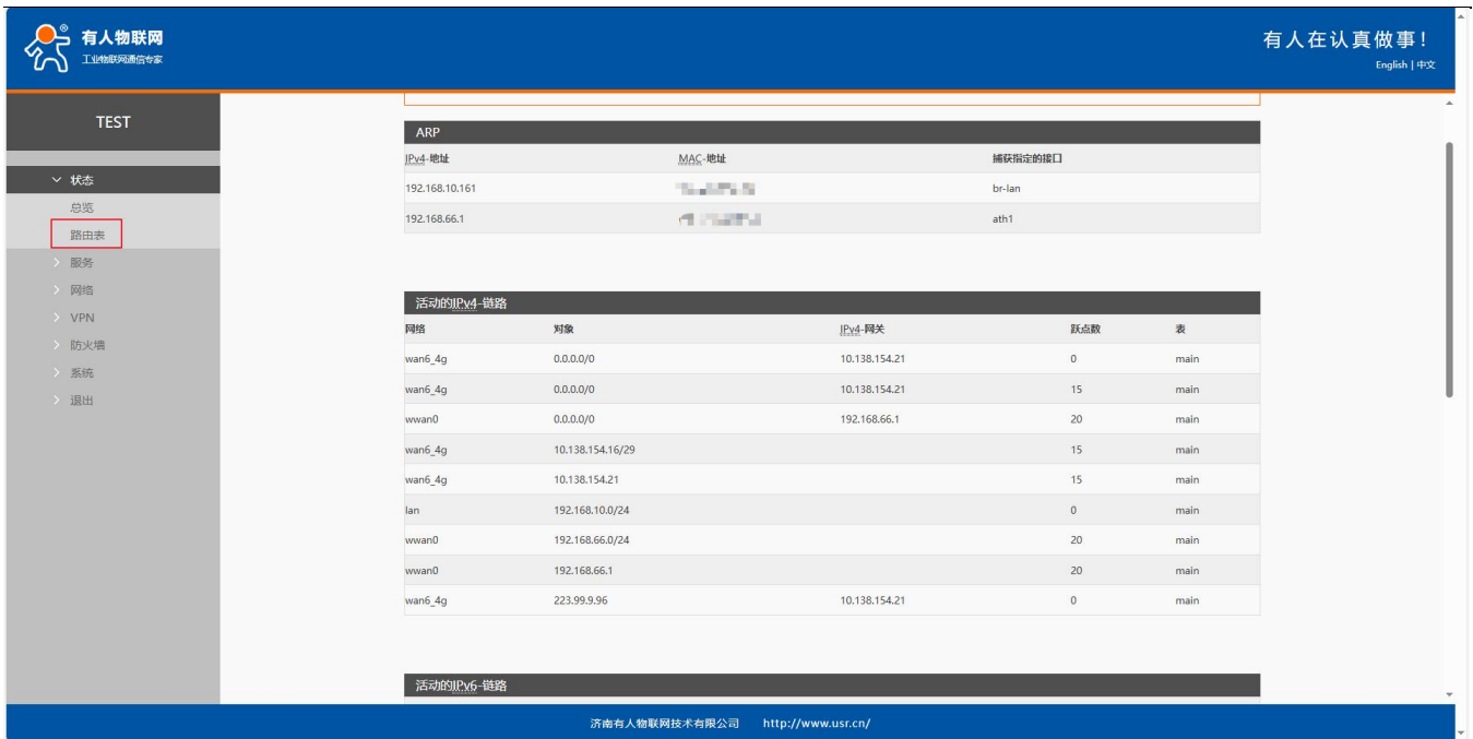
图 5 ARP 表
