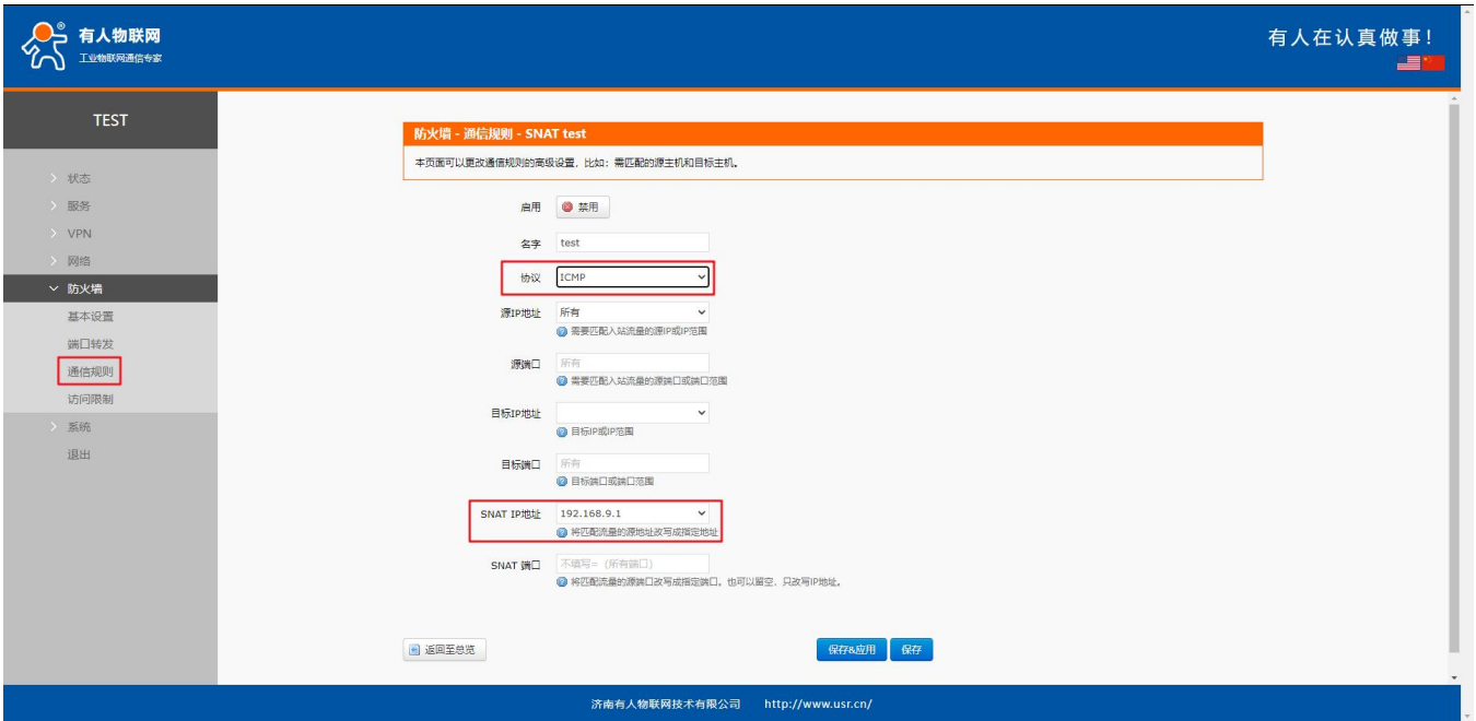
图 82 NAT 设置二
