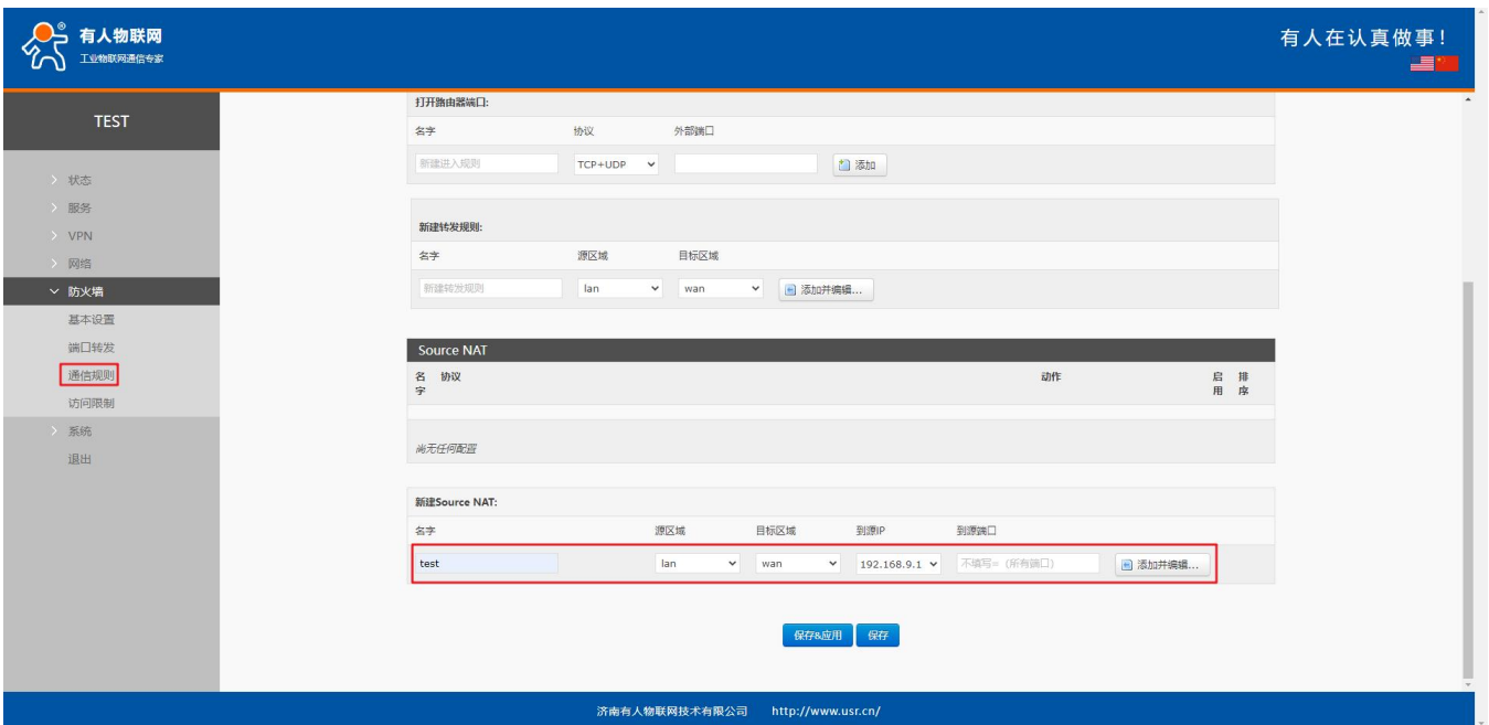
图 81 NAT 设置一
