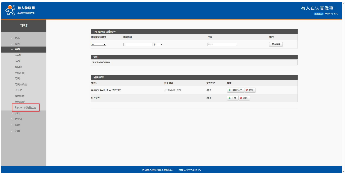
图 43 TCPDUMP
