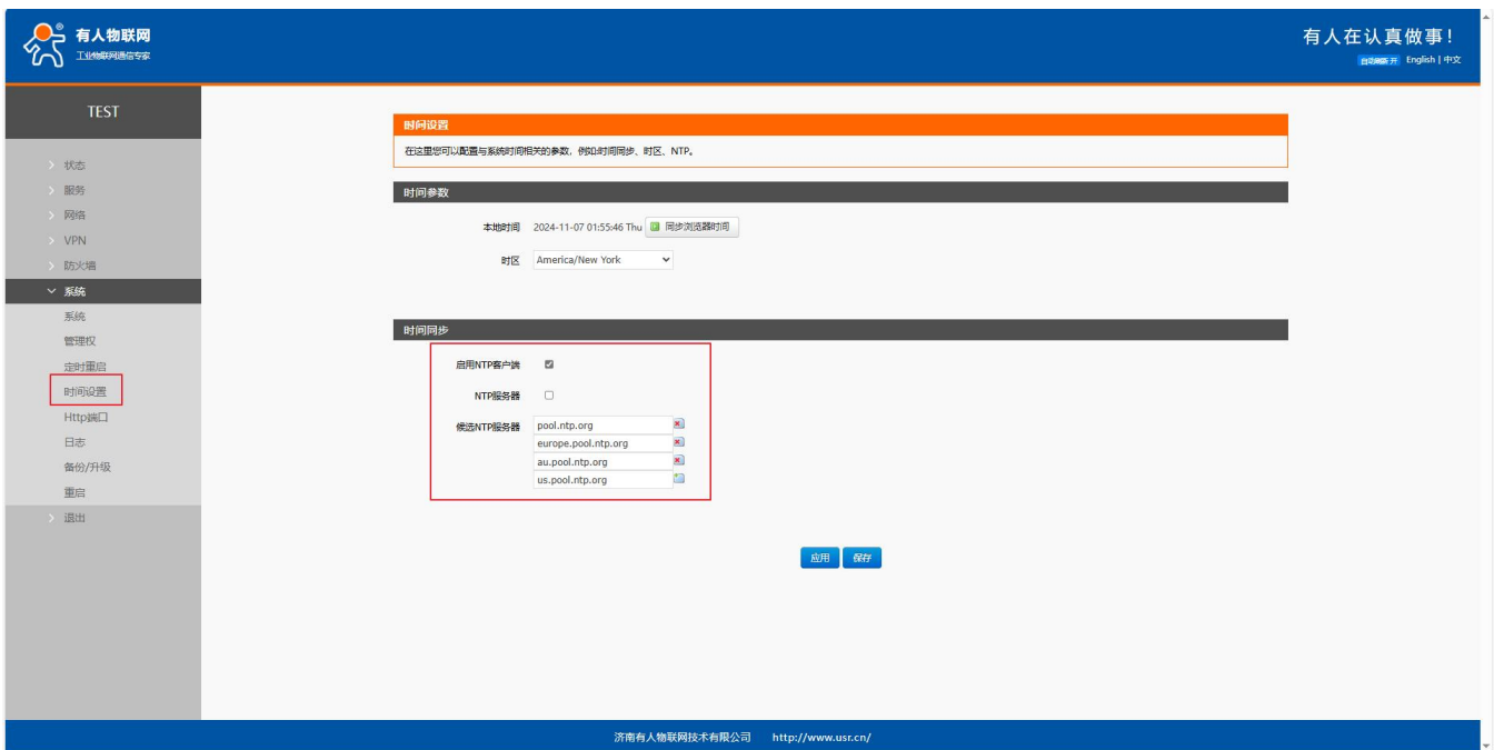
图 102 NTP 页面
