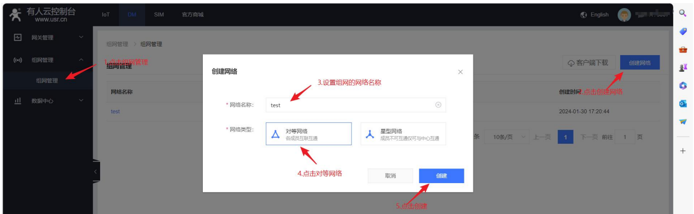
图 8 创建网络
