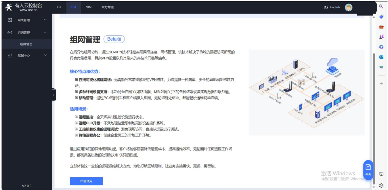
图 7 组网申请
