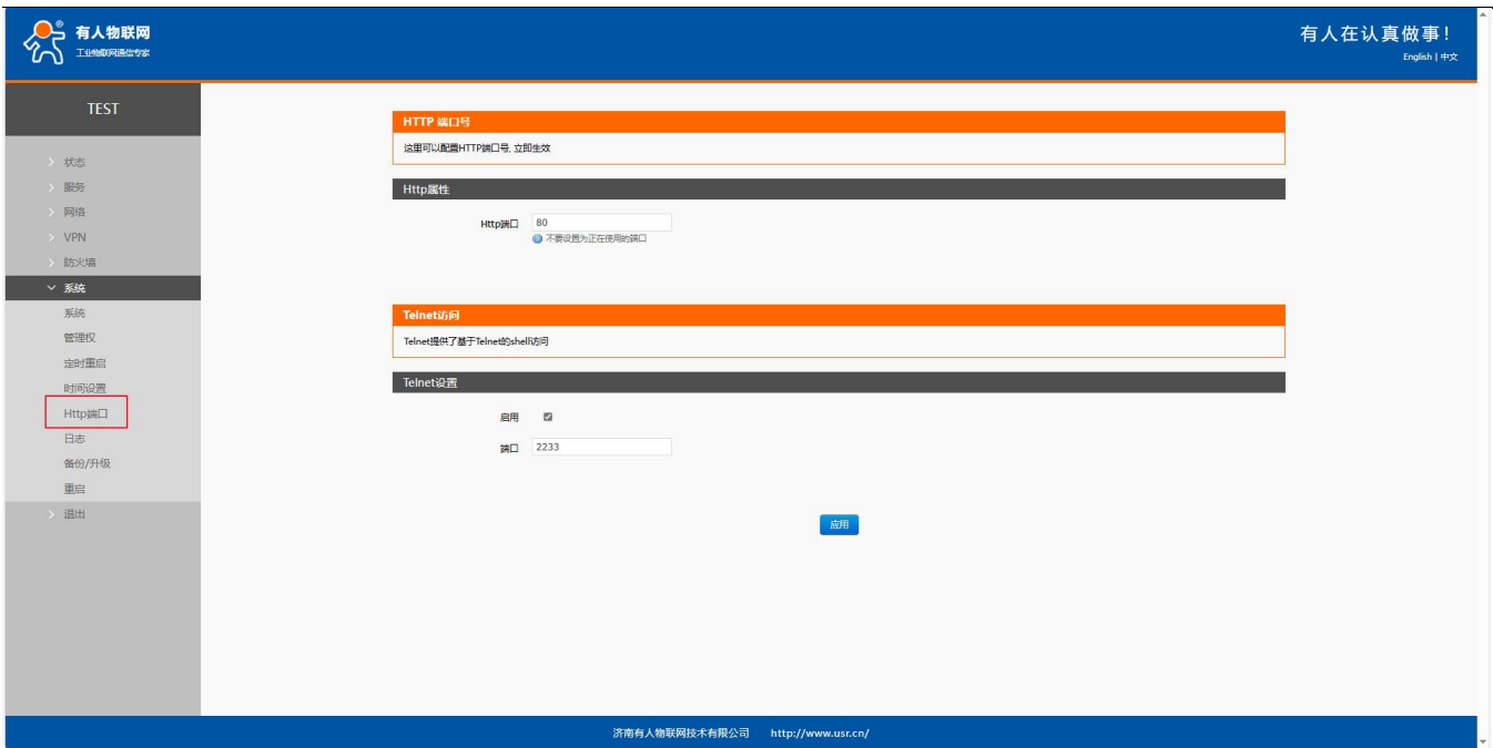
图 104 HTTP 端口
