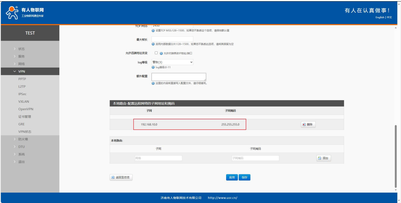
图 65 路由器 2 配置 2
