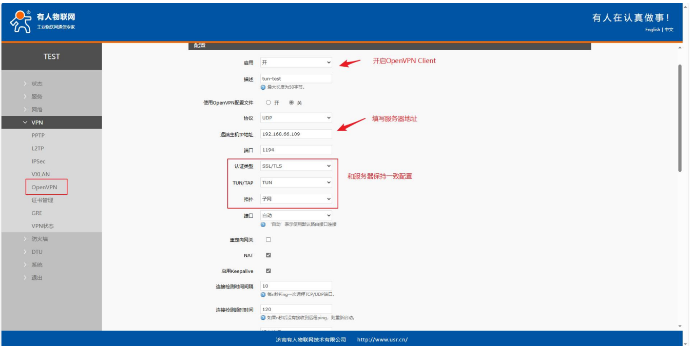
图 64 路由器 2 配置 1
