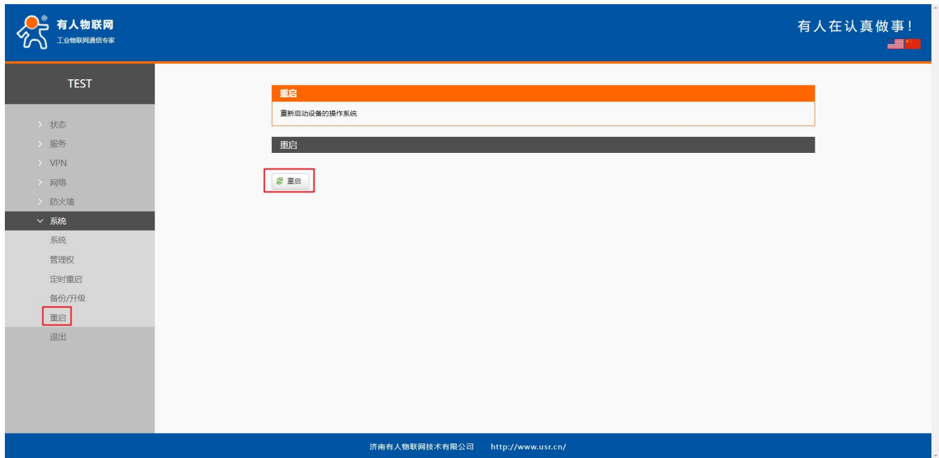
图 108 重启页面
