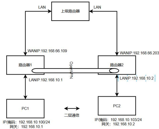
图 50 连接拓扑
