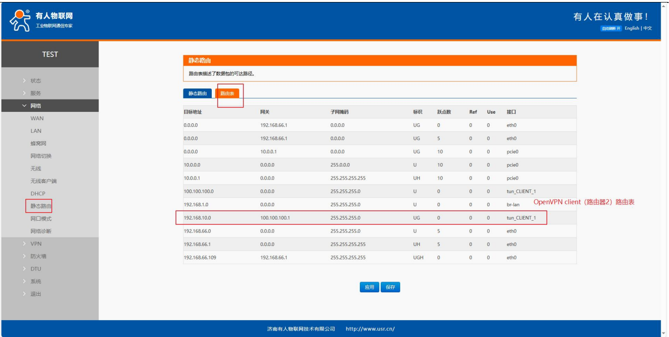
图 68 路由器 2 的路由信息
