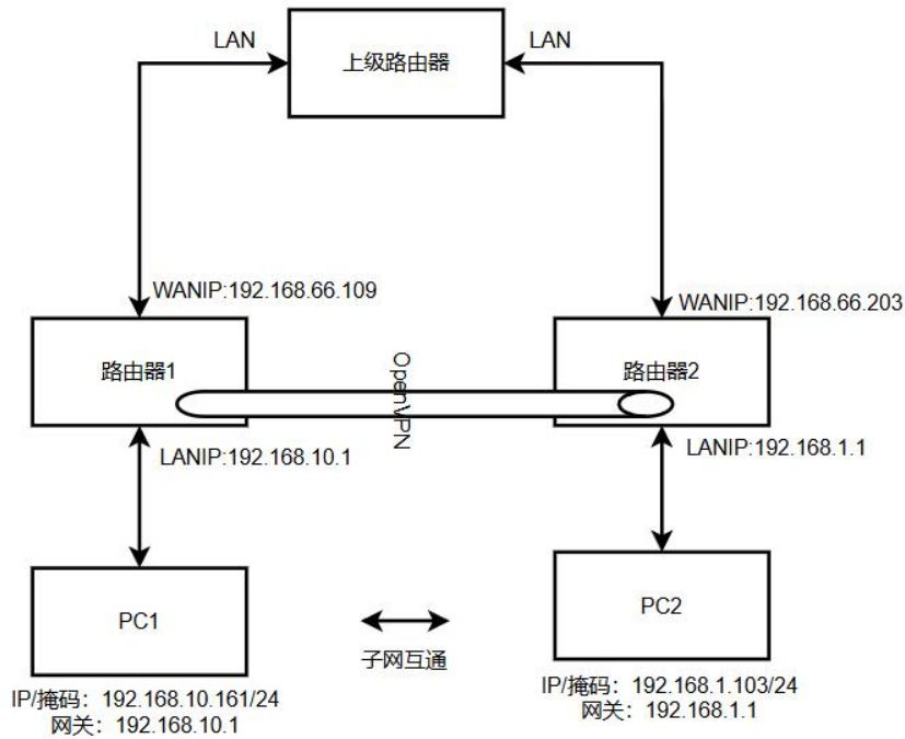
图 59 连接拓扑
