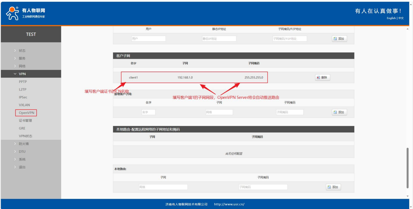
图 62 路由器 1 配置 3
