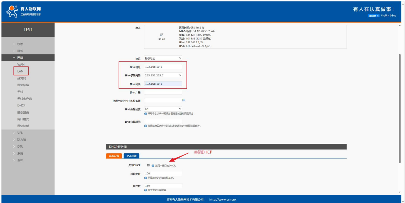
图 51 LAN 口配置
