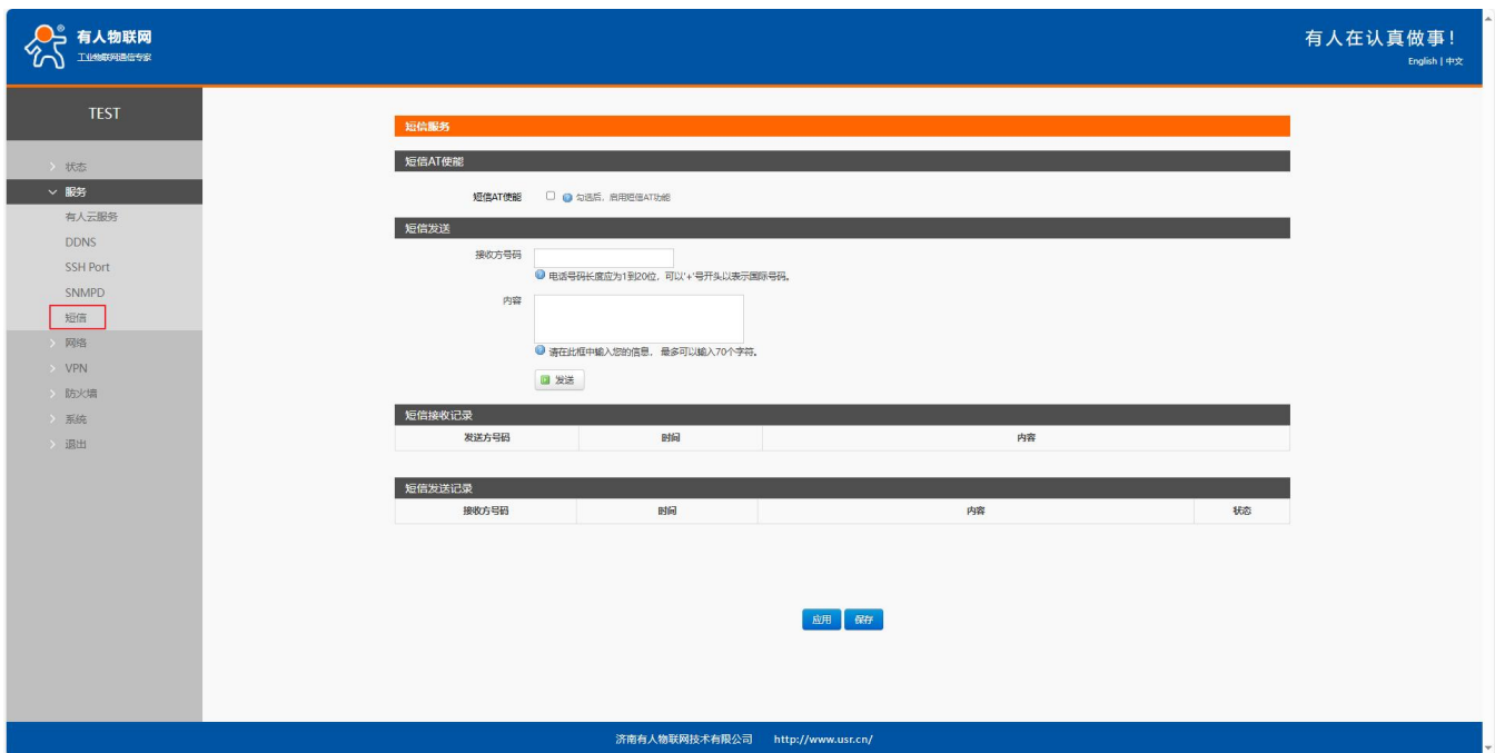
图 97 短信
