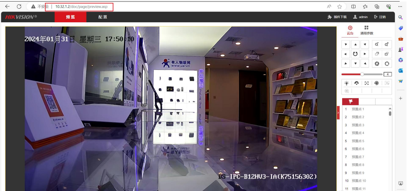
图 19 远程监控
