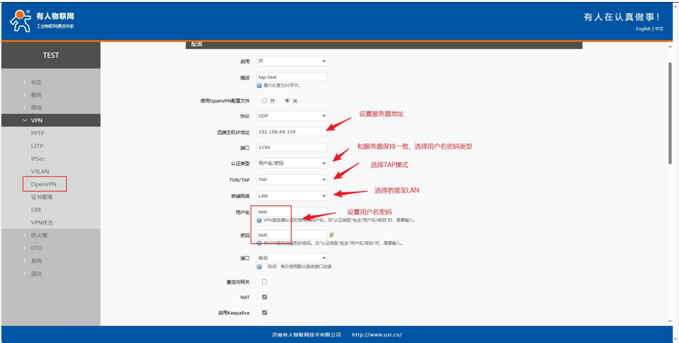
图 56 openvpn 配置 1
