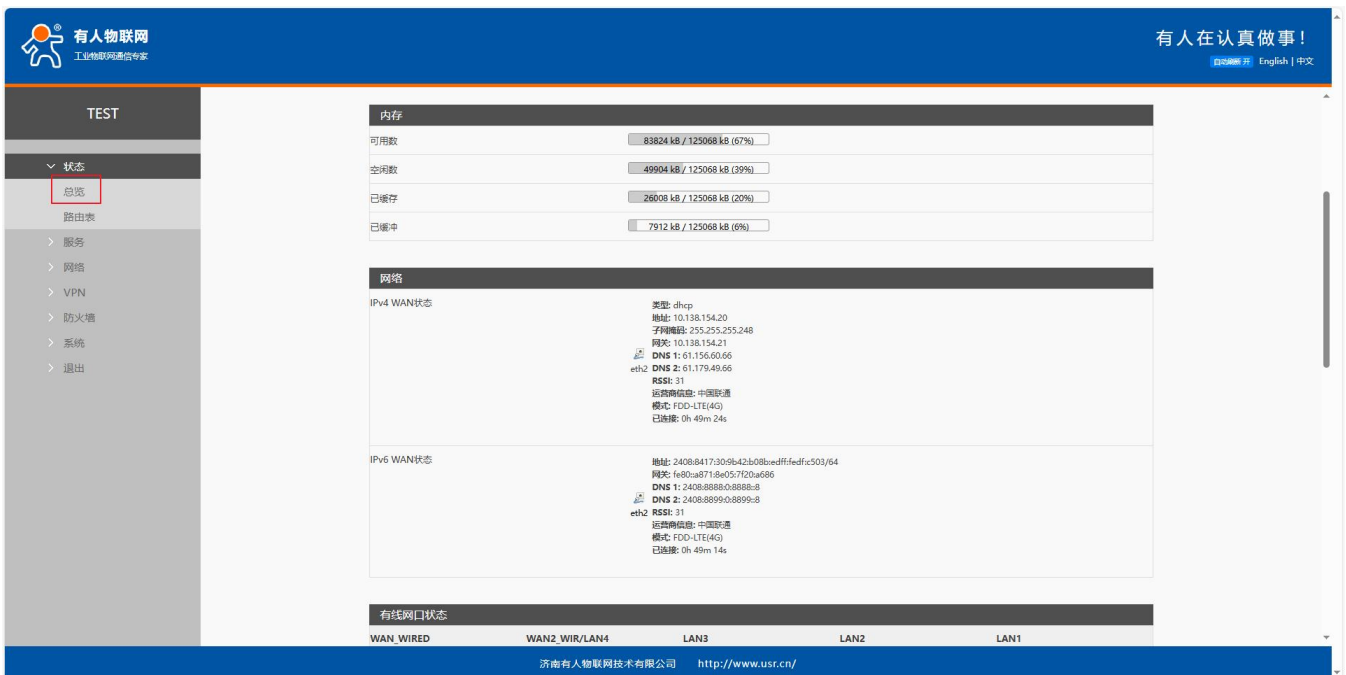
图 4 状态总览
