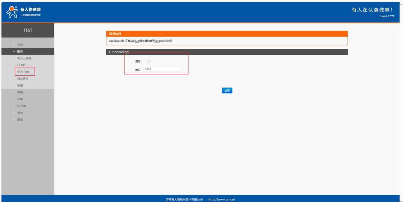
图 96 SSH
