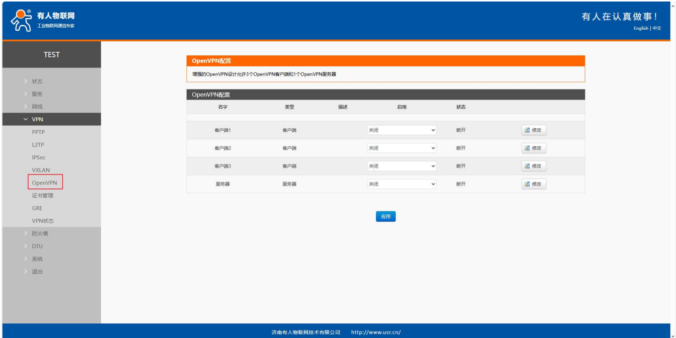
图 48 OpenVPN 页面
