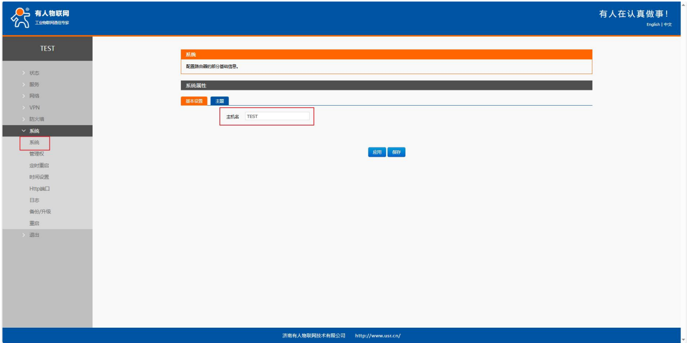
图 101 主机名
