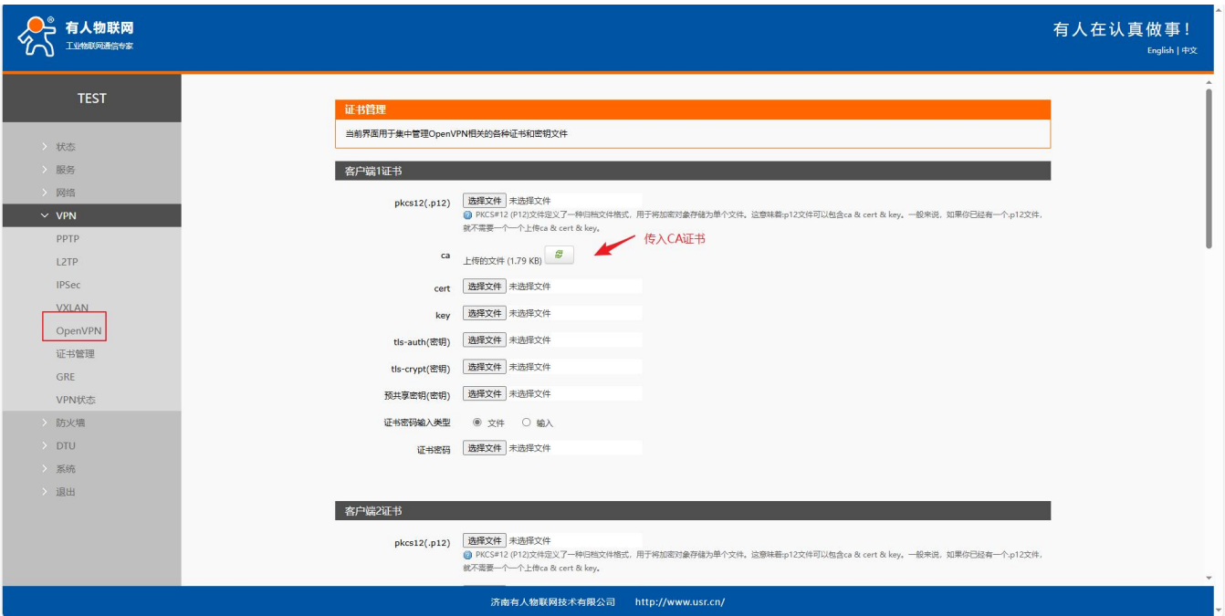
图 57 Openvpn 配置 2
