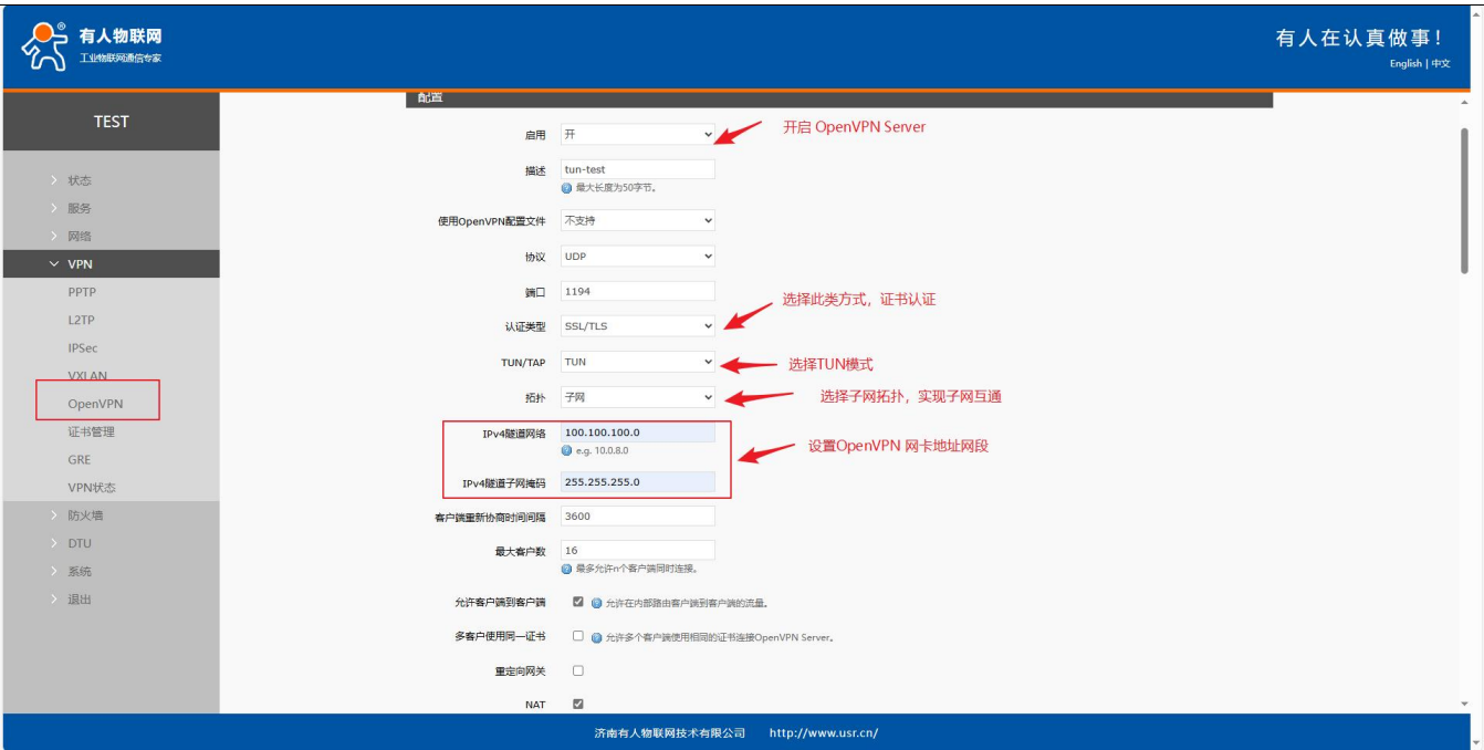
图 61 路由器 1 配置 2
