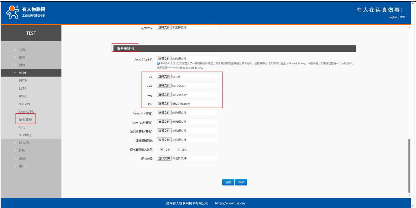
图 63 路由器 1 配置 4
