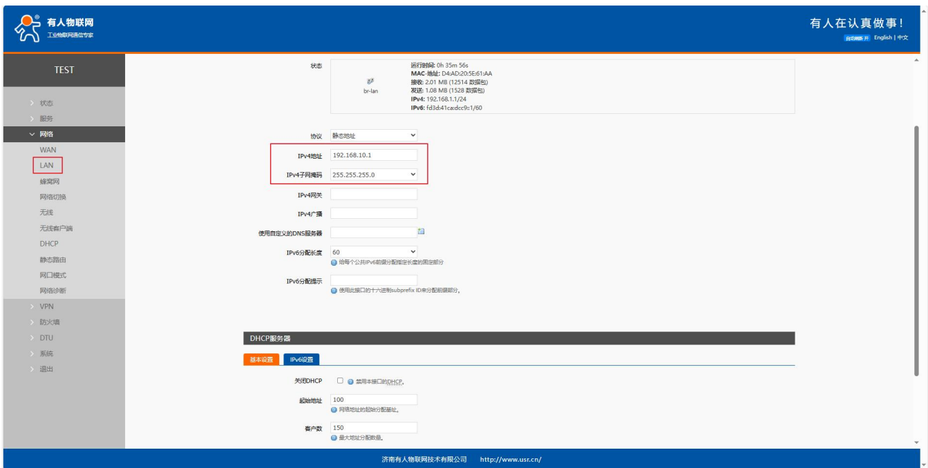
图 60 路由器 1 配置 1
