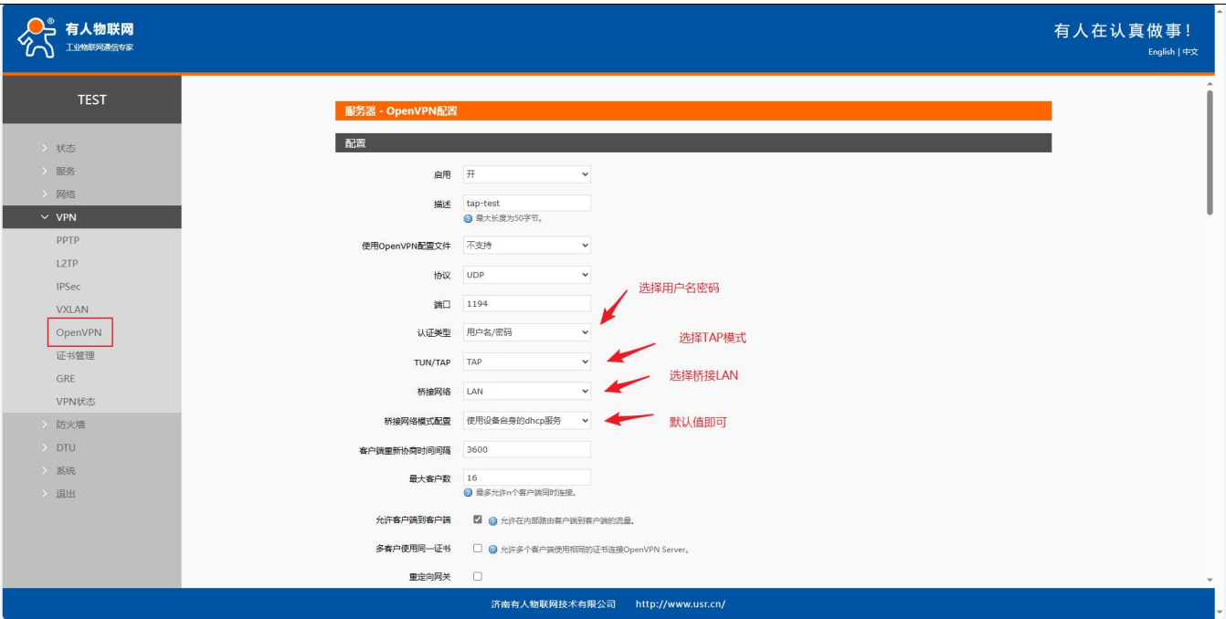
图 52 Openvpn 配置 1
