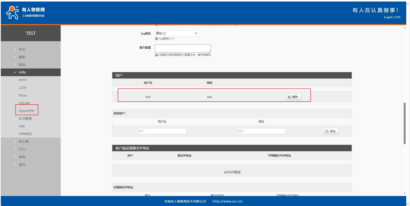
图 53 Openvpn 配置 2
