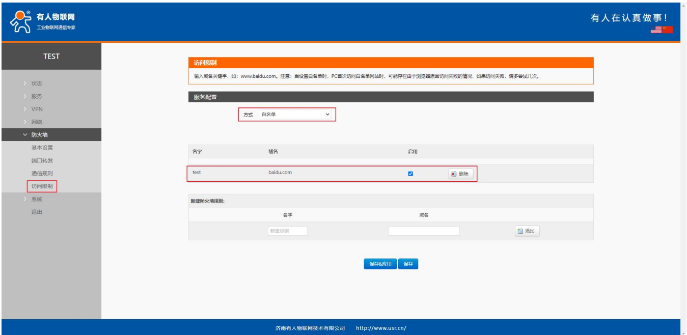
图 90 域名白名单
