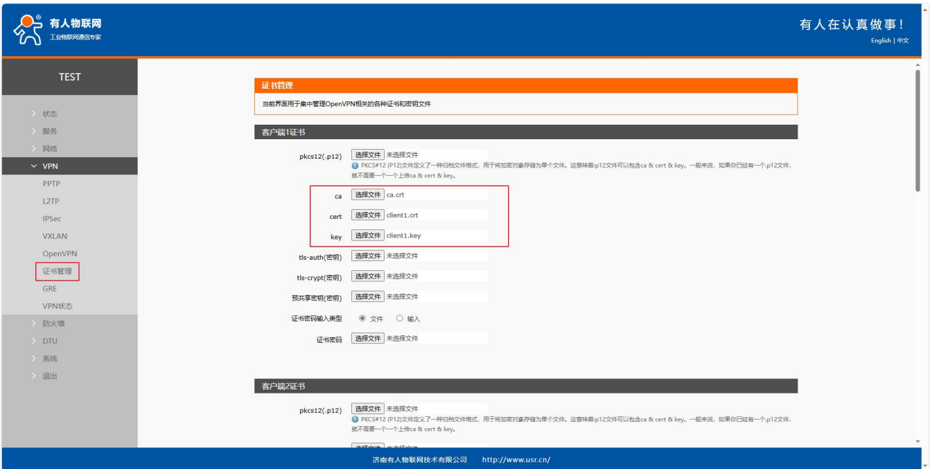
图 66 路由器 2 配置 3
