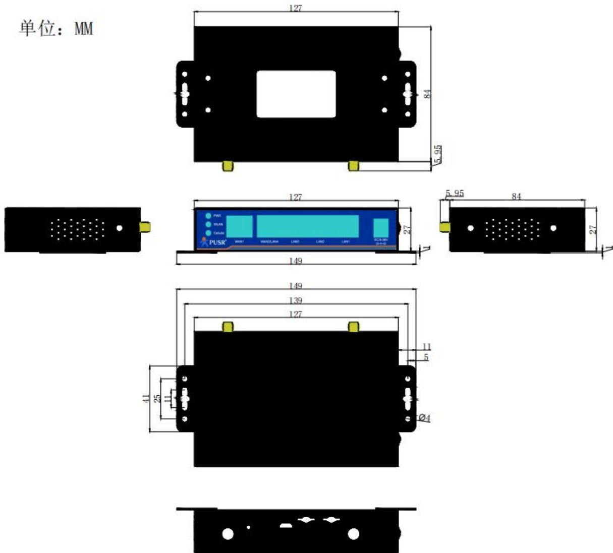
图 2 USR-G805 外观尺寸图
