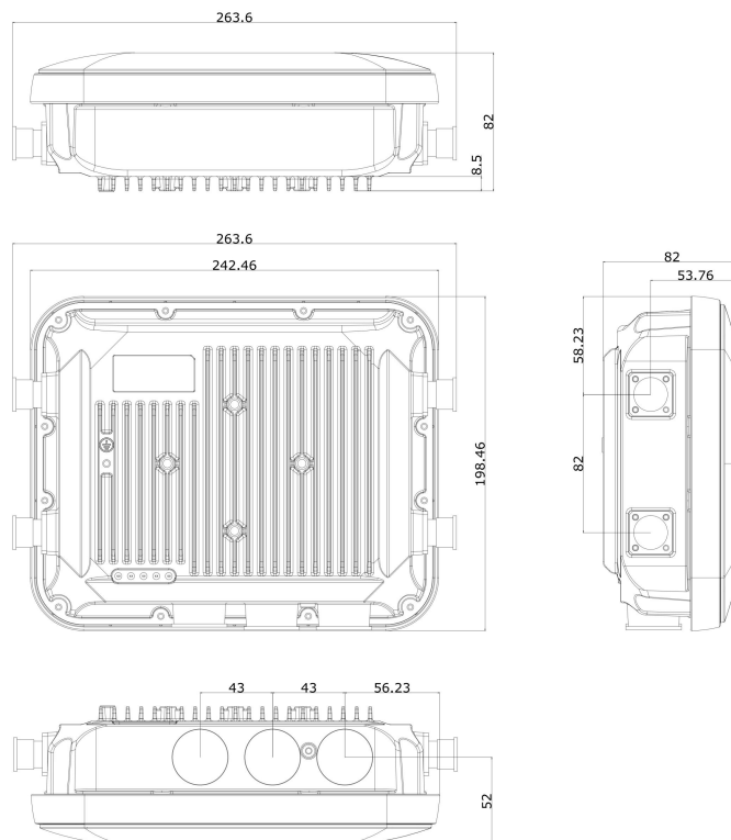
图 1 AP520X 尺寸图
