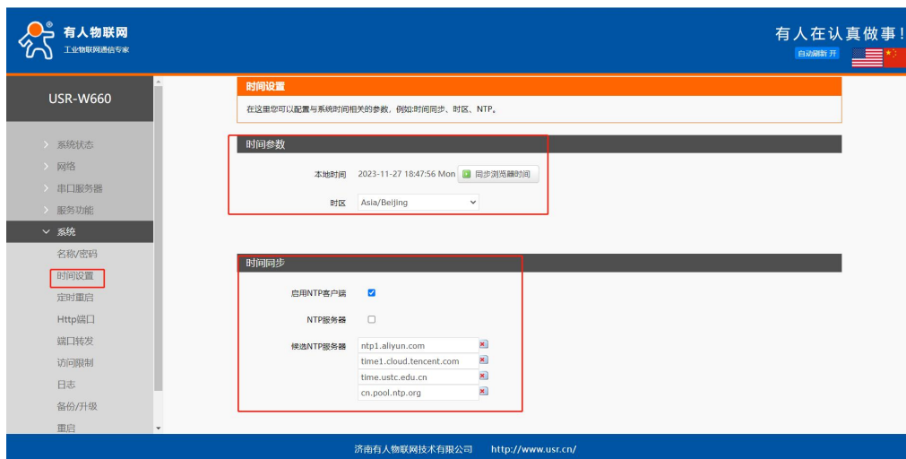
图 65 时区与本地时间同步设置
