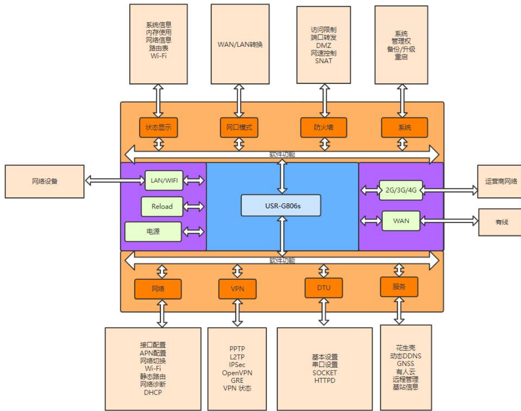
图 3 功能框图
