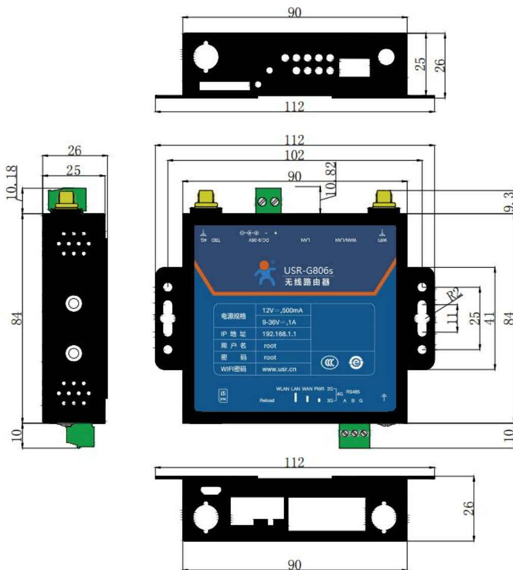
图 1 USR-G806s 尺寸图
