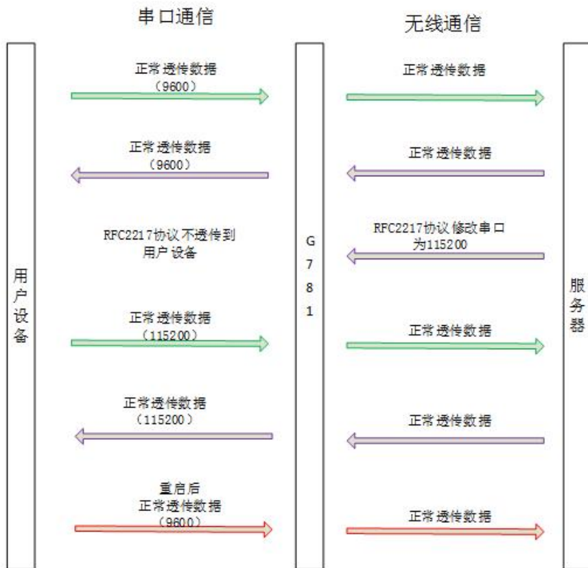
图 114 类 RFC2217 功能示意图
