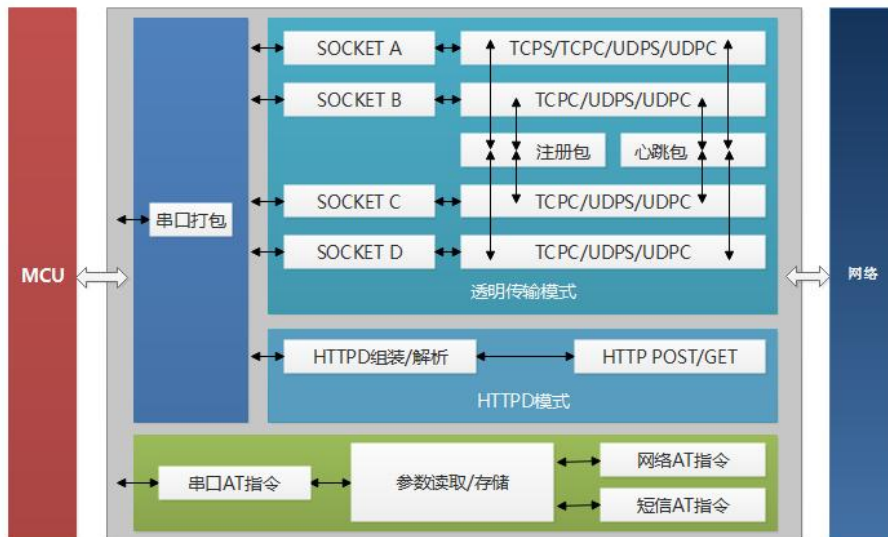
图 105 DTU 功能框图
