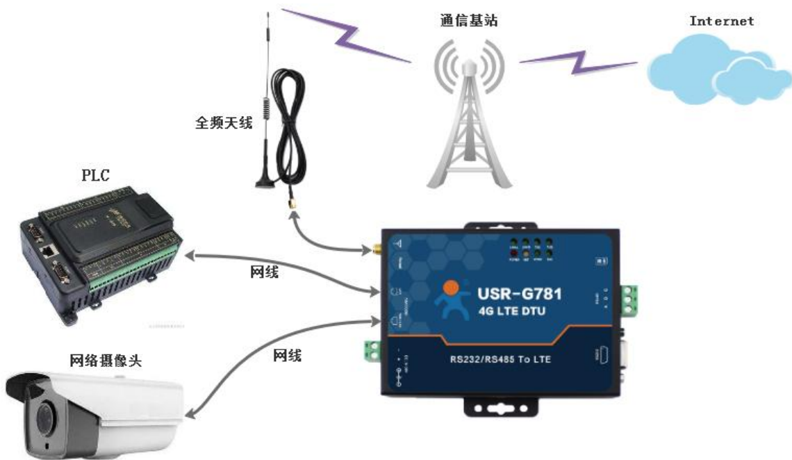
图 103 联网示意图
