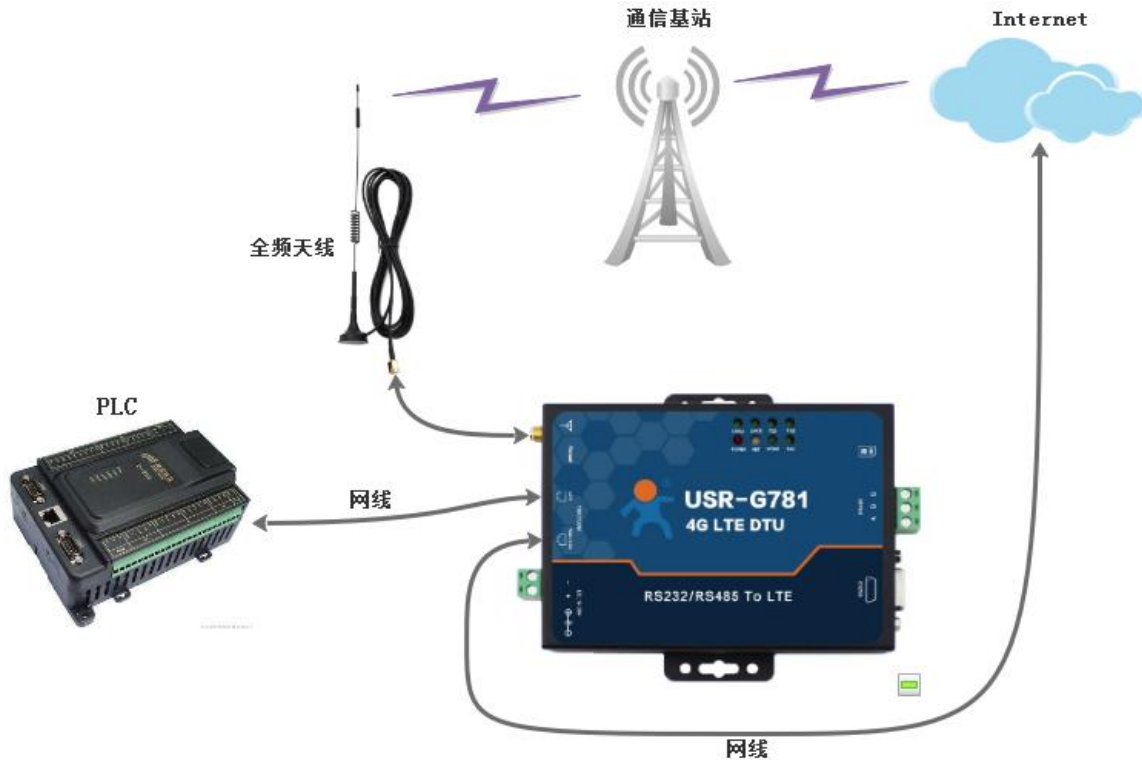
图 101 联网示意图
