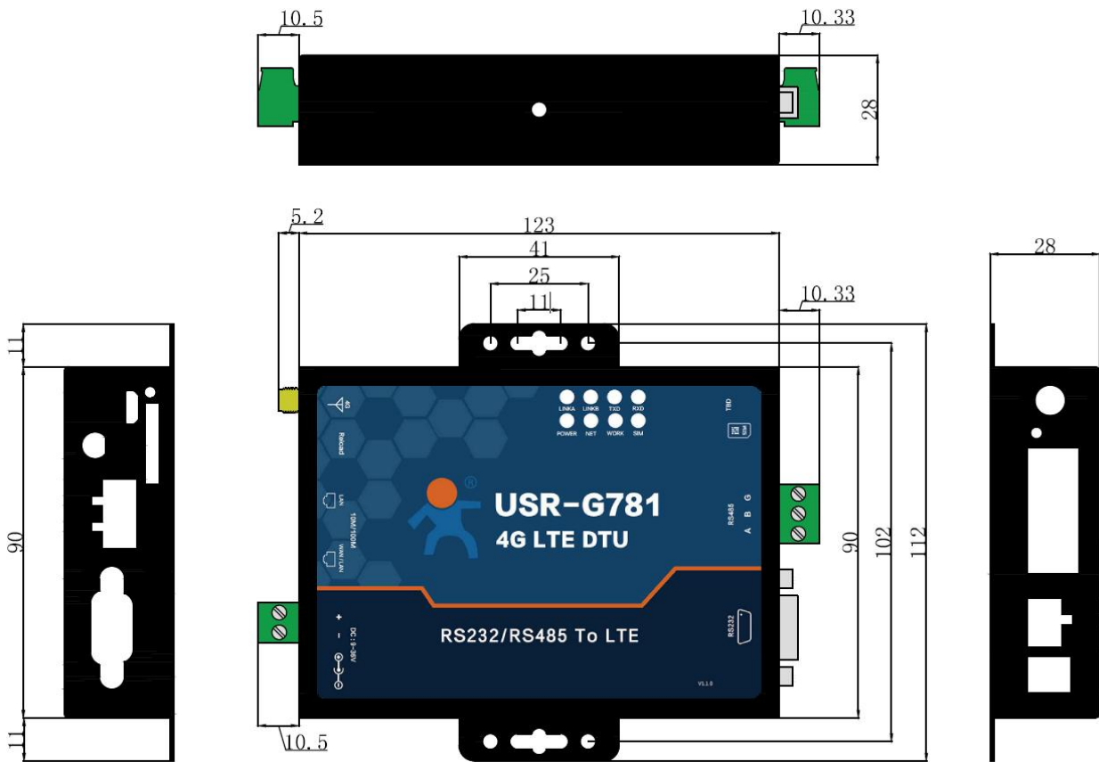
图 2 尺寸示意图
