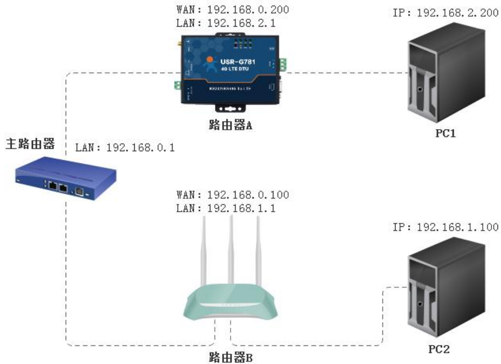
图 35 静态路由表实例图
