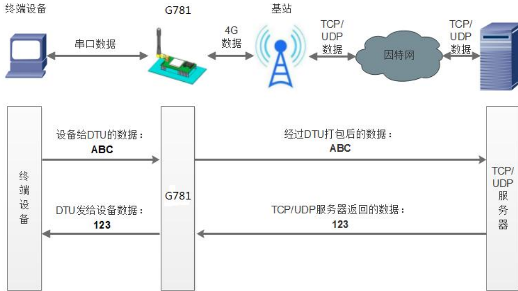
图 106 网络透传模式
