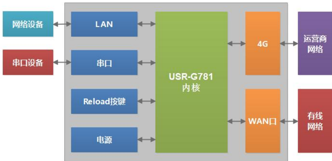
图 3 路由器功能框图
