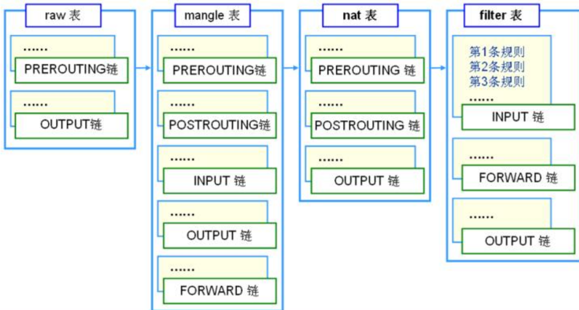
图 74 Linux 系统 iptables 概念框图
