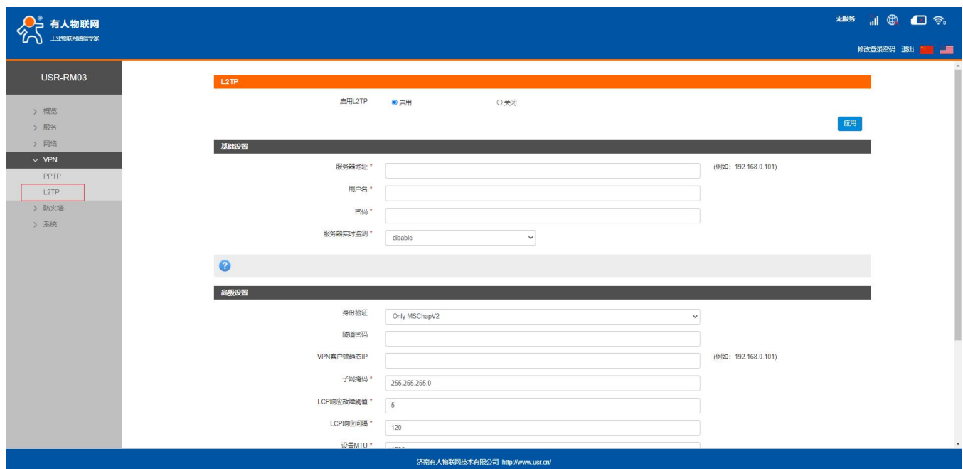
图 42 L2TP 基本设置
