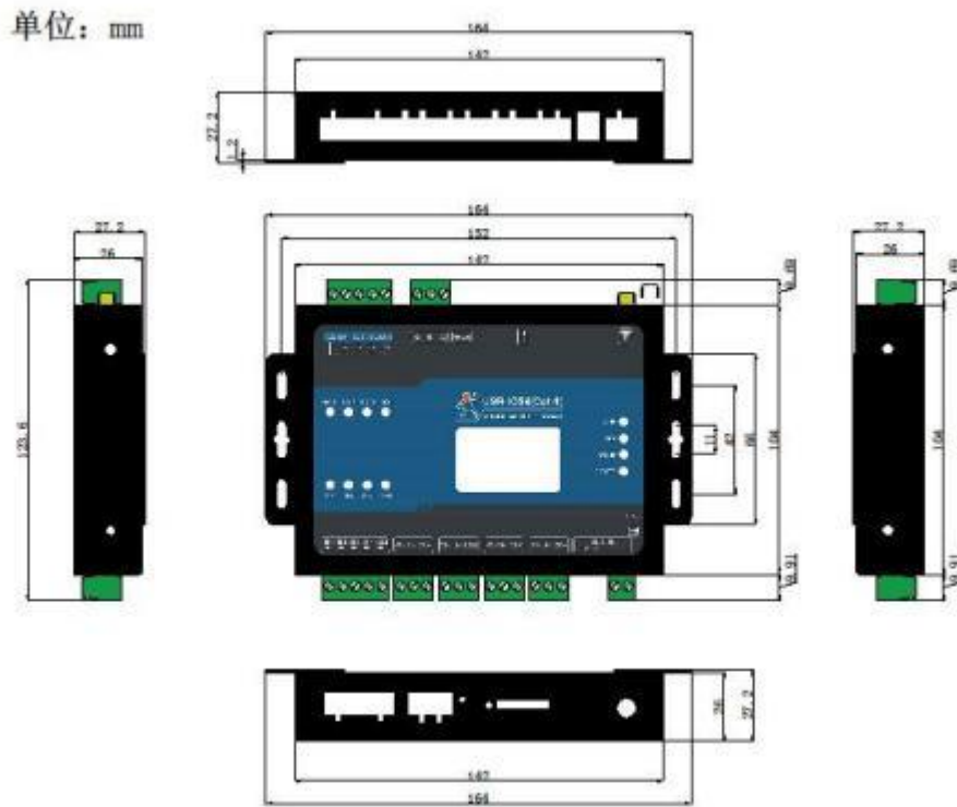
图 15 USR-IO34-CAT1 尺寸图
