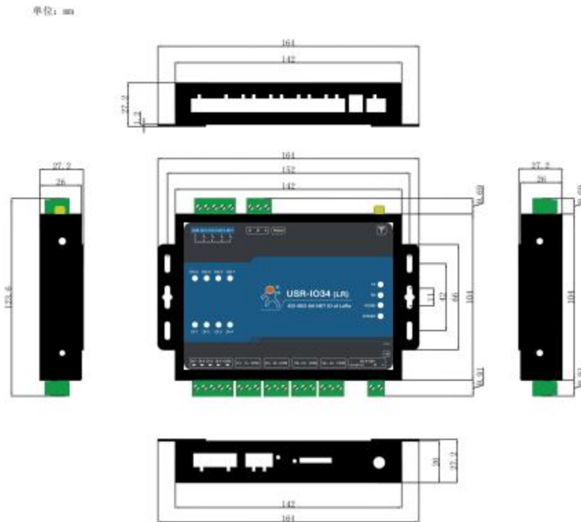
图 24 USR-IO34-LR-C 尺寸图
