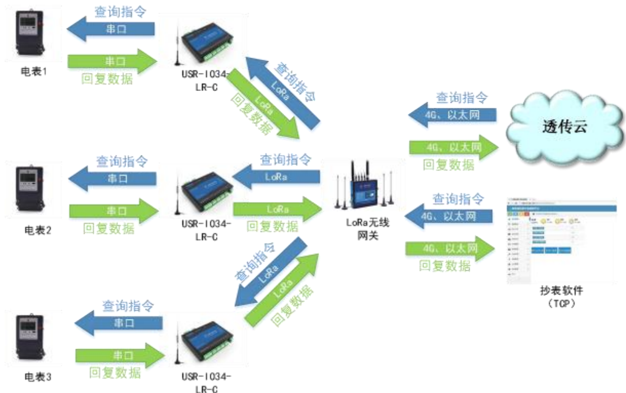
图 32 Modbus 数据采集系统示意图
