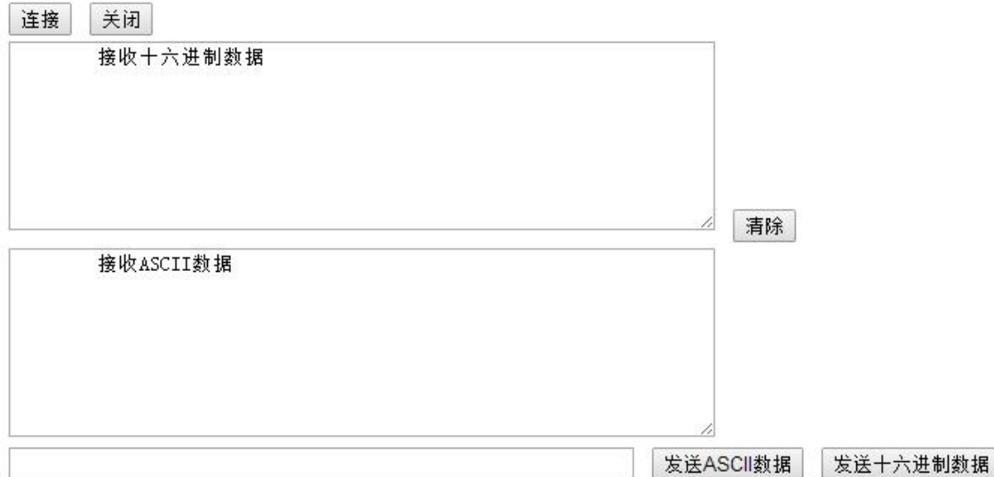
图 36 WebSocket 页面
