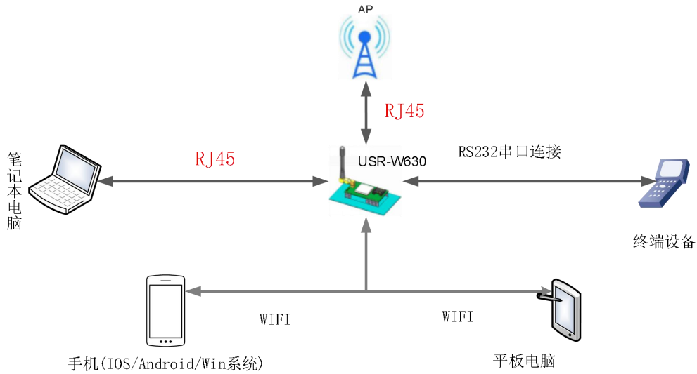
图 5 网线桥接应用场景
