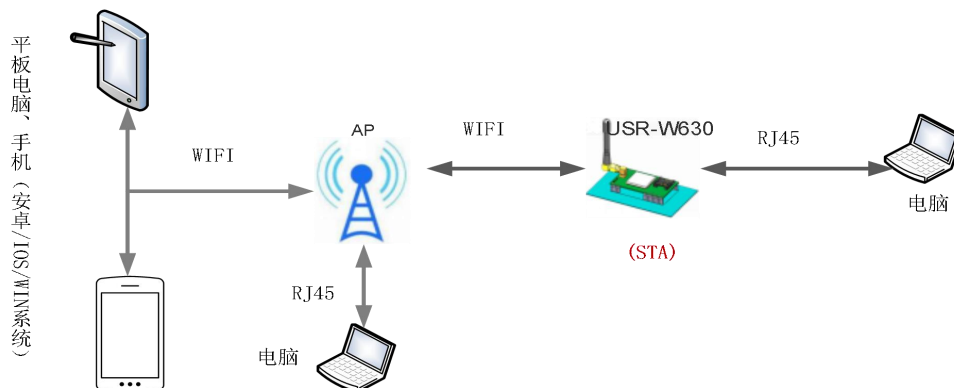
图 8 有线加无线的应用场景 2
