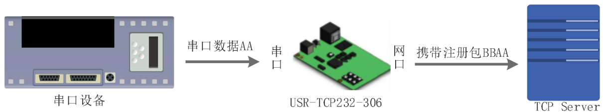
图 29 数据携带注册包
