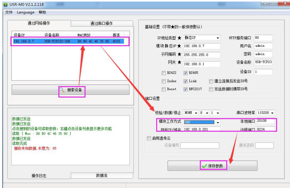
图 15 UDP Client 软件设置
