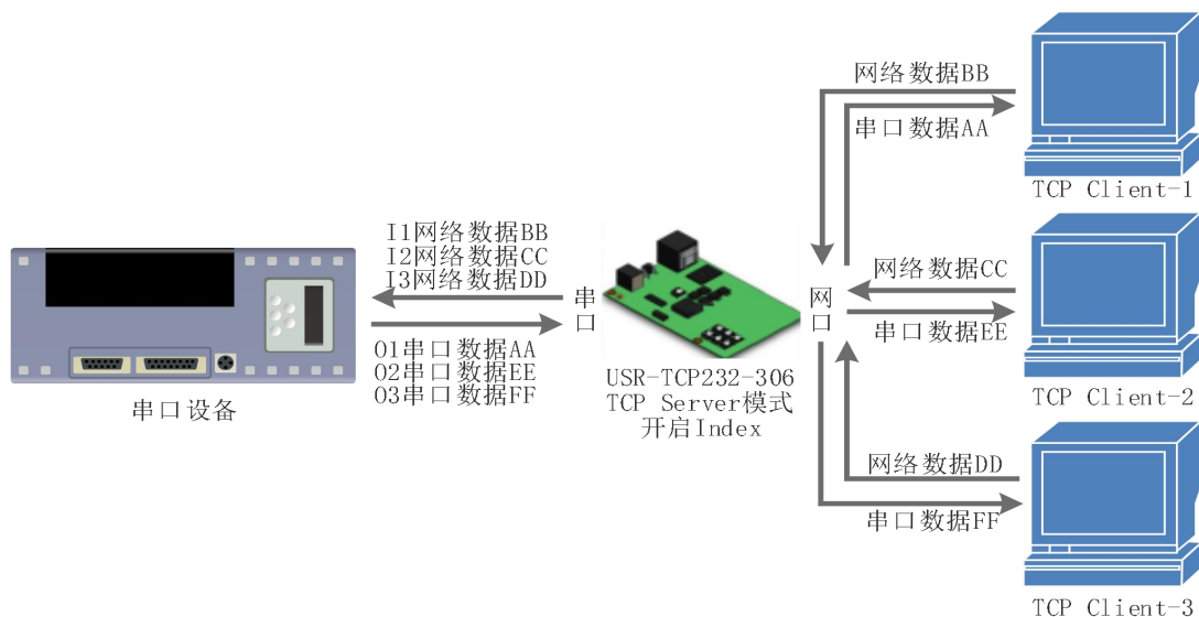
图 35 Index 功能示意图
