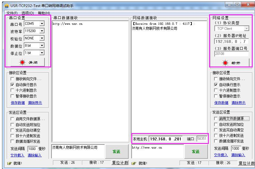
图 13 TCP Server 透传测试
