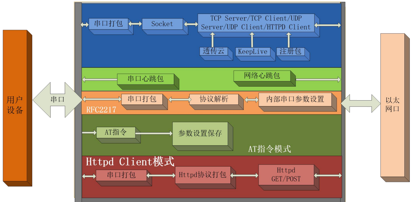
306 功能框图
