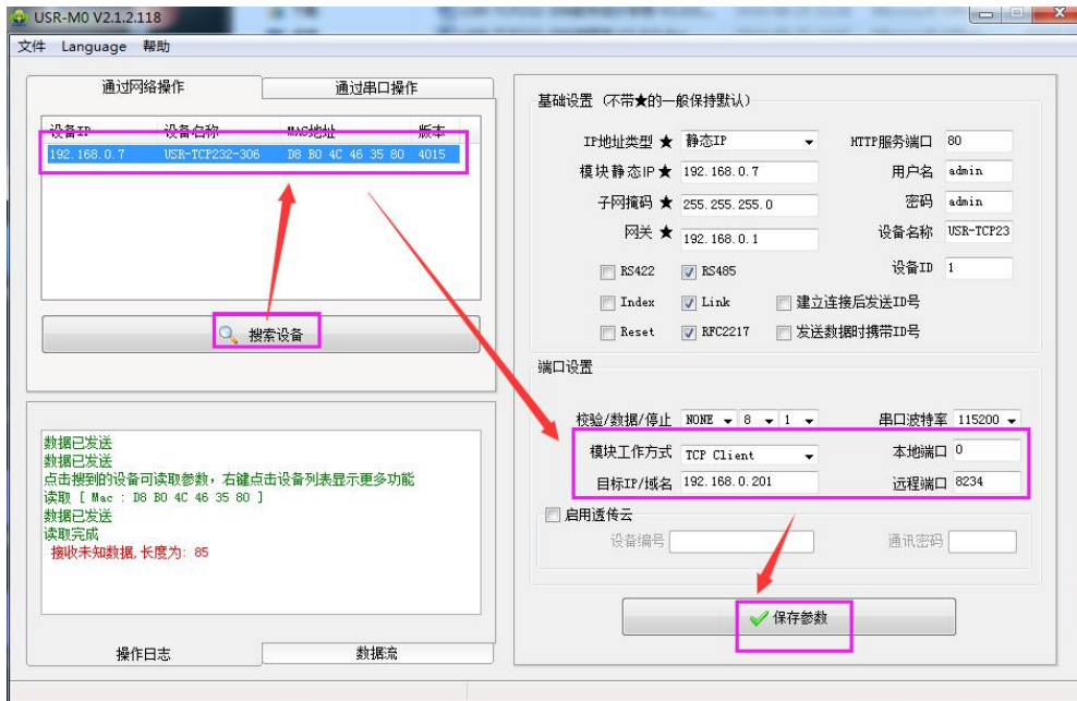
图 7 TCP Client 软件设置
