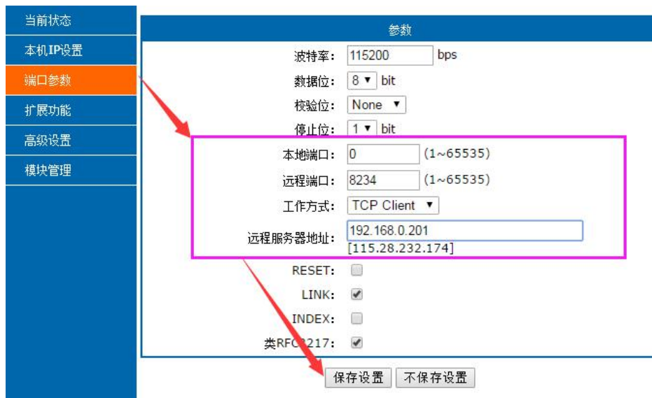
图 8 TCP Client 网页设置
