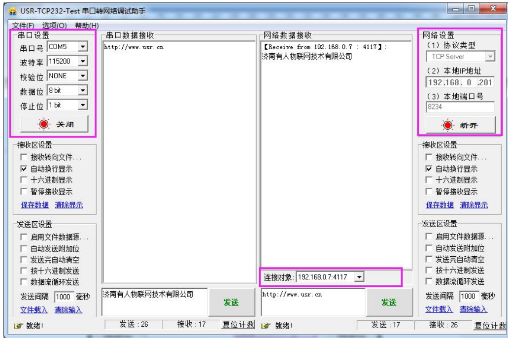
图 9 TCP Client 透传测试
