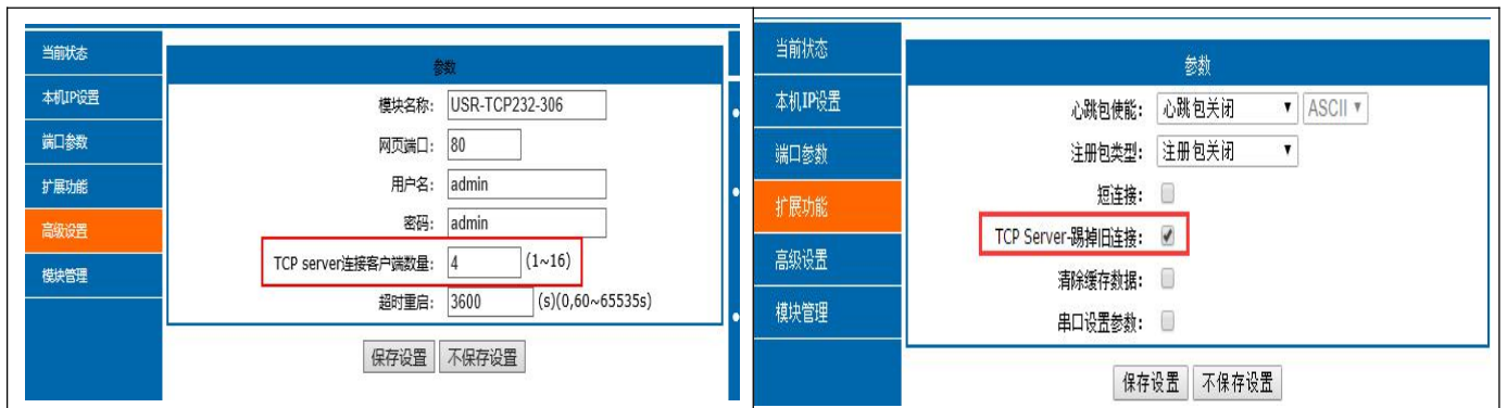
图 37 TCP Server 连接 Client 最大值与踢掉旧连接设置
