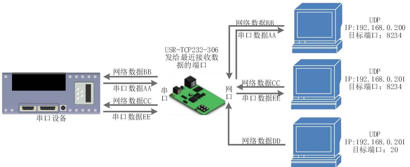
图 18 UDP Server 模式说明
