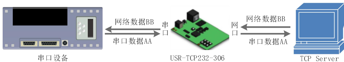
图 6 TCP Client 模式说明
