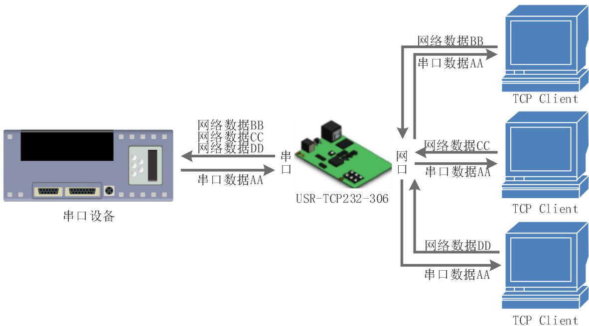
图 10 TCP Server 模式说明
