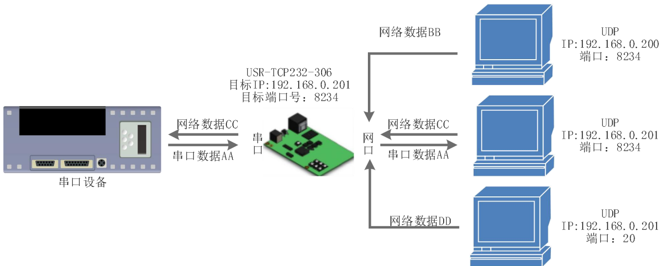
图 14 UDP Client 模式说明
