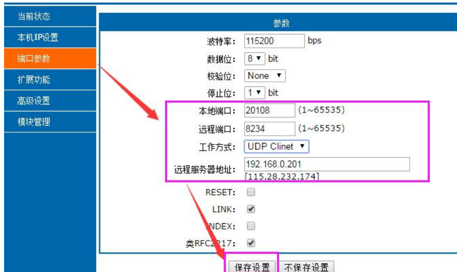
图 16 UDP Client 网页设置
