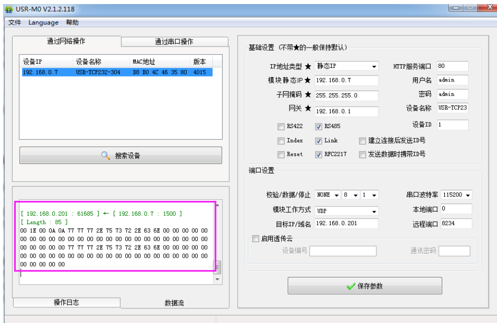
图 42. 抓取报文示例
