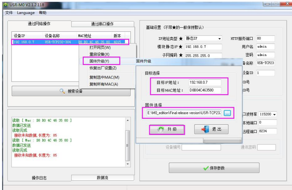
图 5. 选择固件
