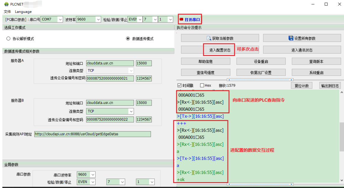
图 8 进入串口 AT 指令模式
