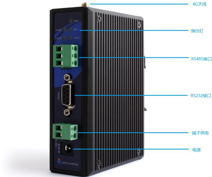
图 1 产品外观
