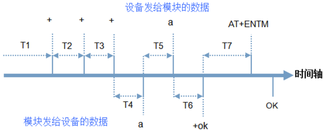
图7 模式切换时序图
