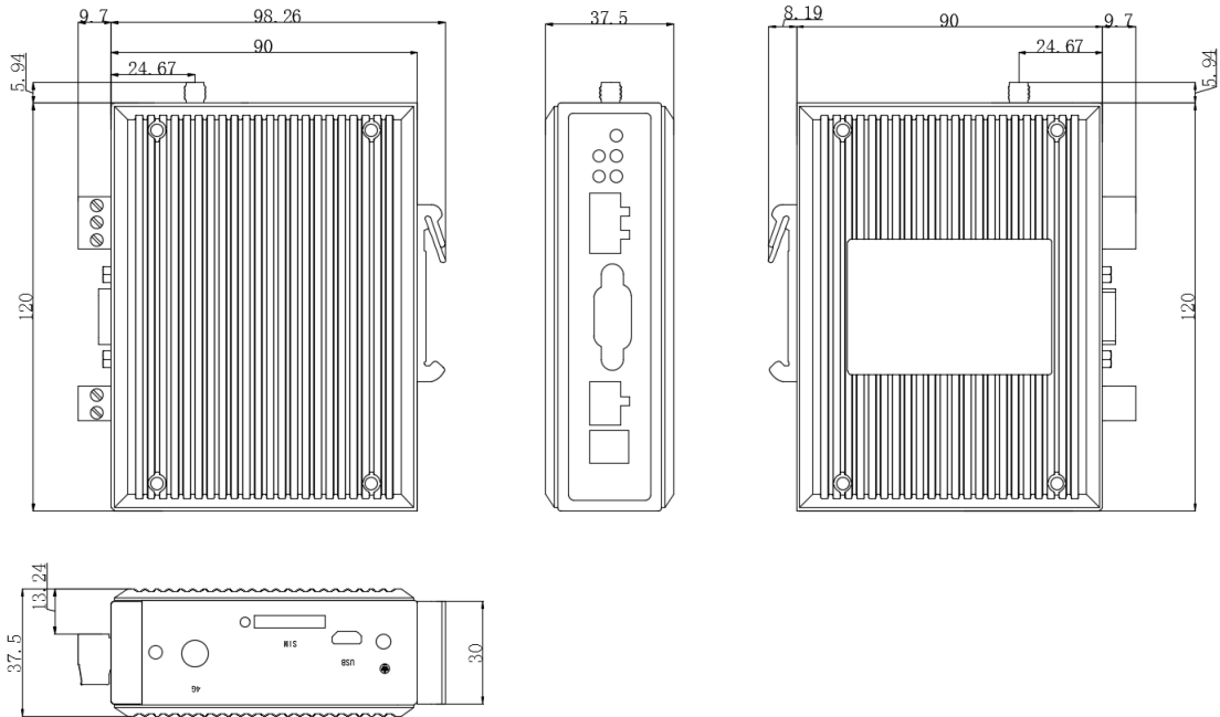
图 2 PLCNET300 尺寸图
