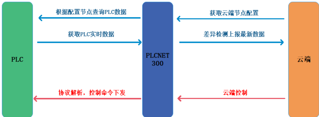
图 4 协议解析模式示意图
