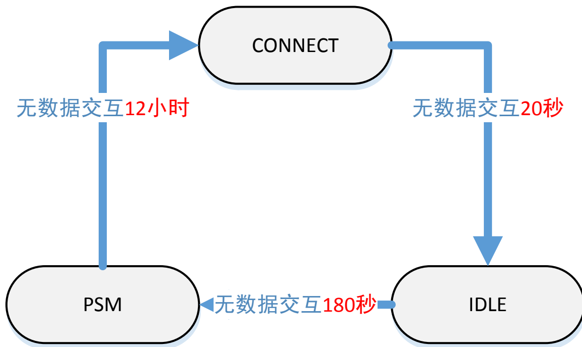
图 10 网络连接状态切换示意图
