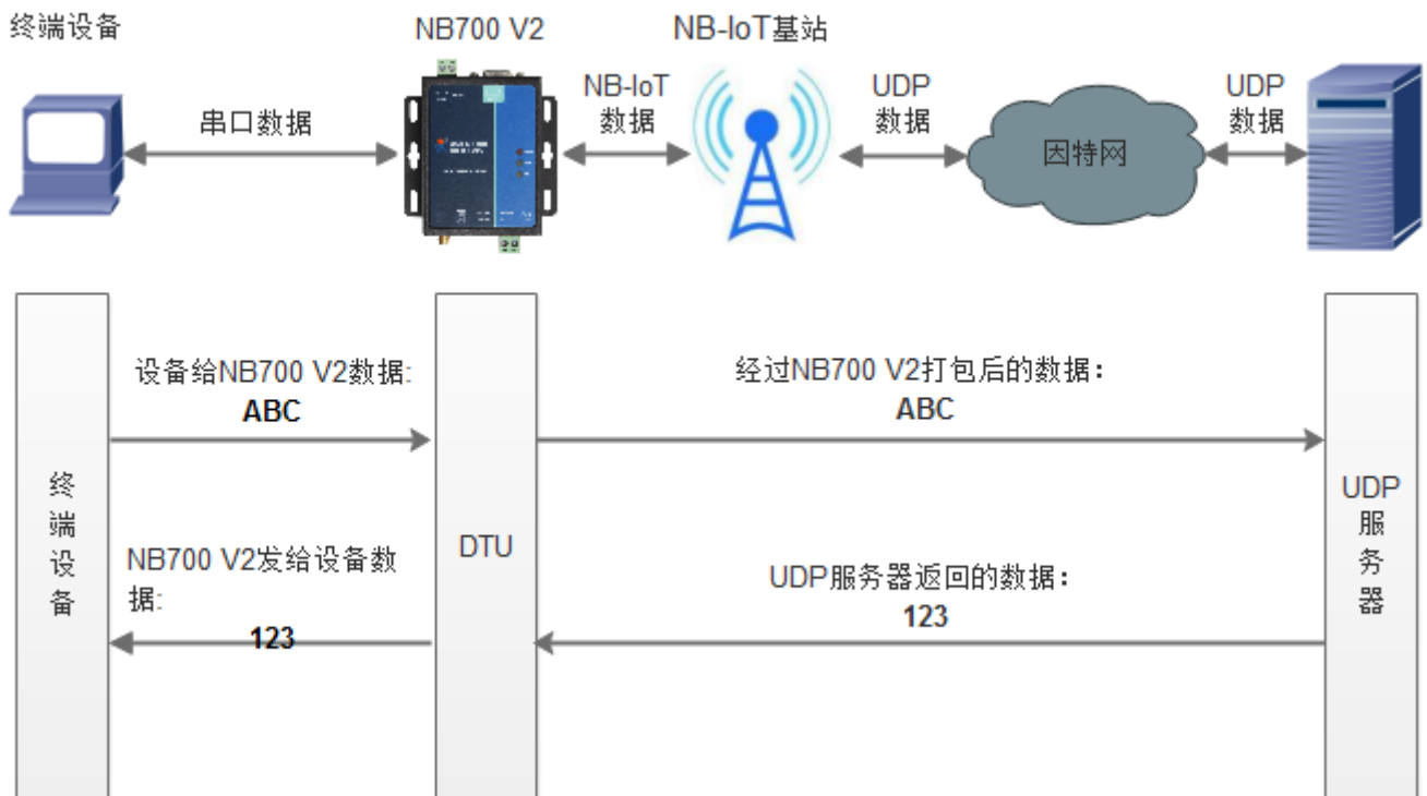
图 2 网络透传模式示意图
