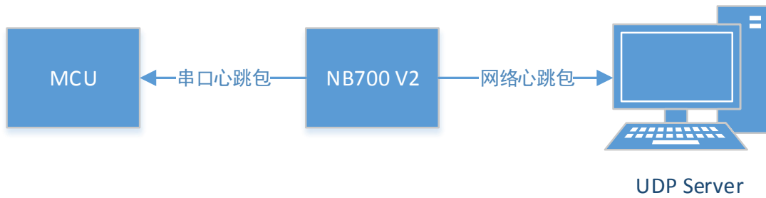
图 13 心跳包功能示意图
