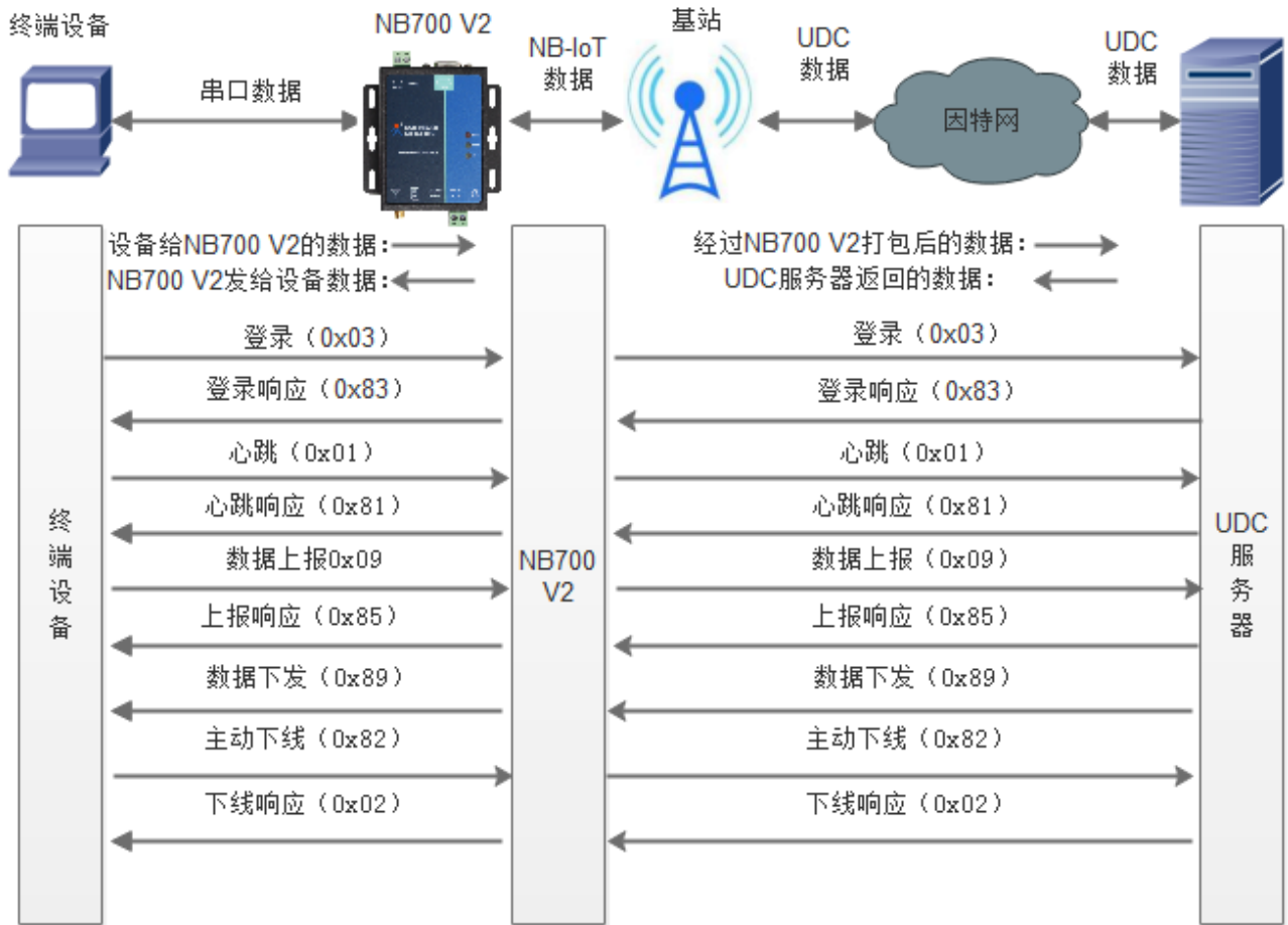
图 6 协议透传 UDC 模式示意图
