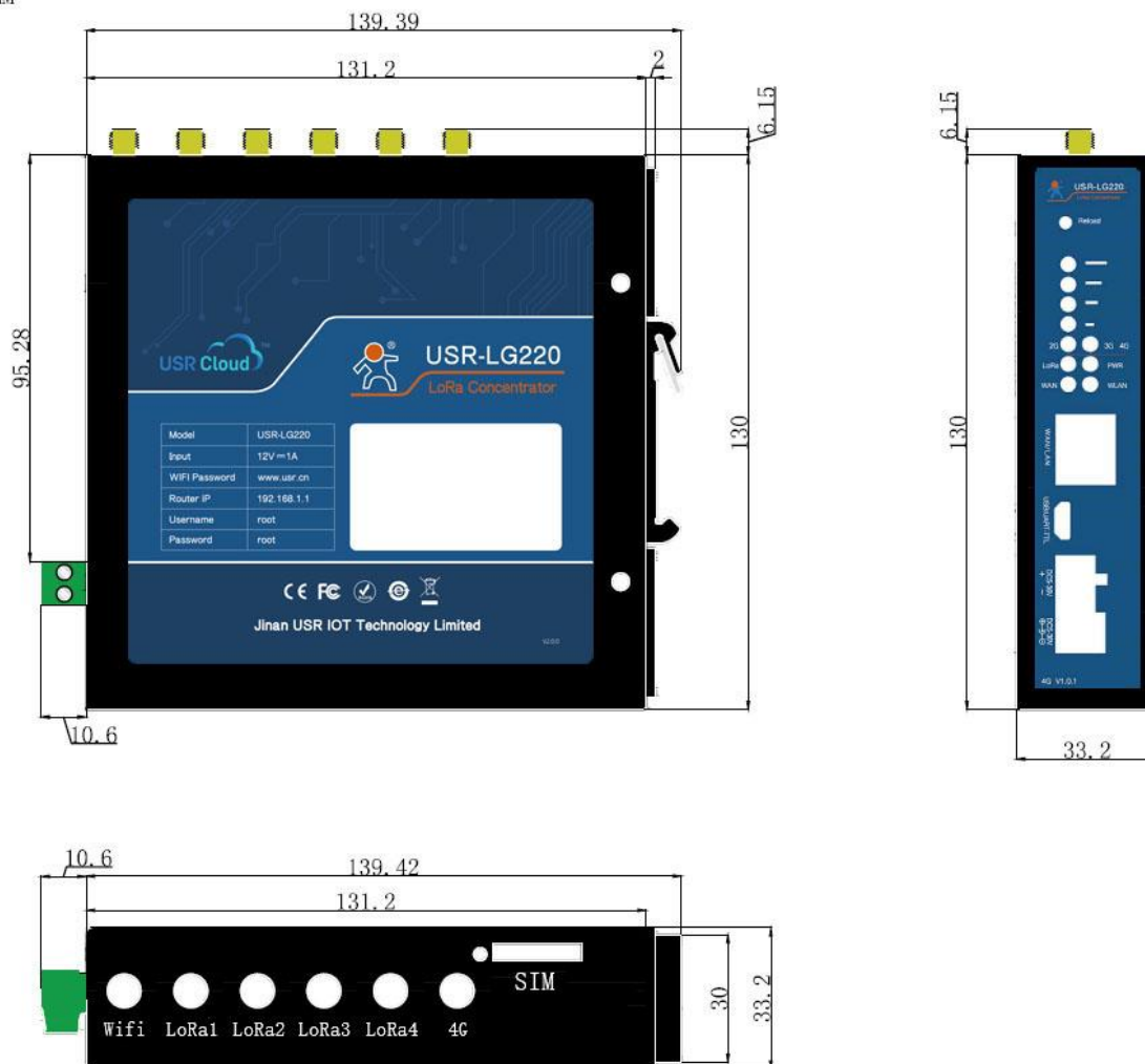
图 2 USR-LG220-L 尺寸示意图
