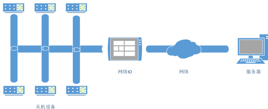
图 28 主机模式联网应用示意
