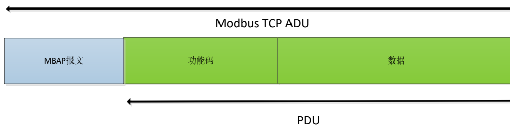
图 38 Modbus TCP 帧
