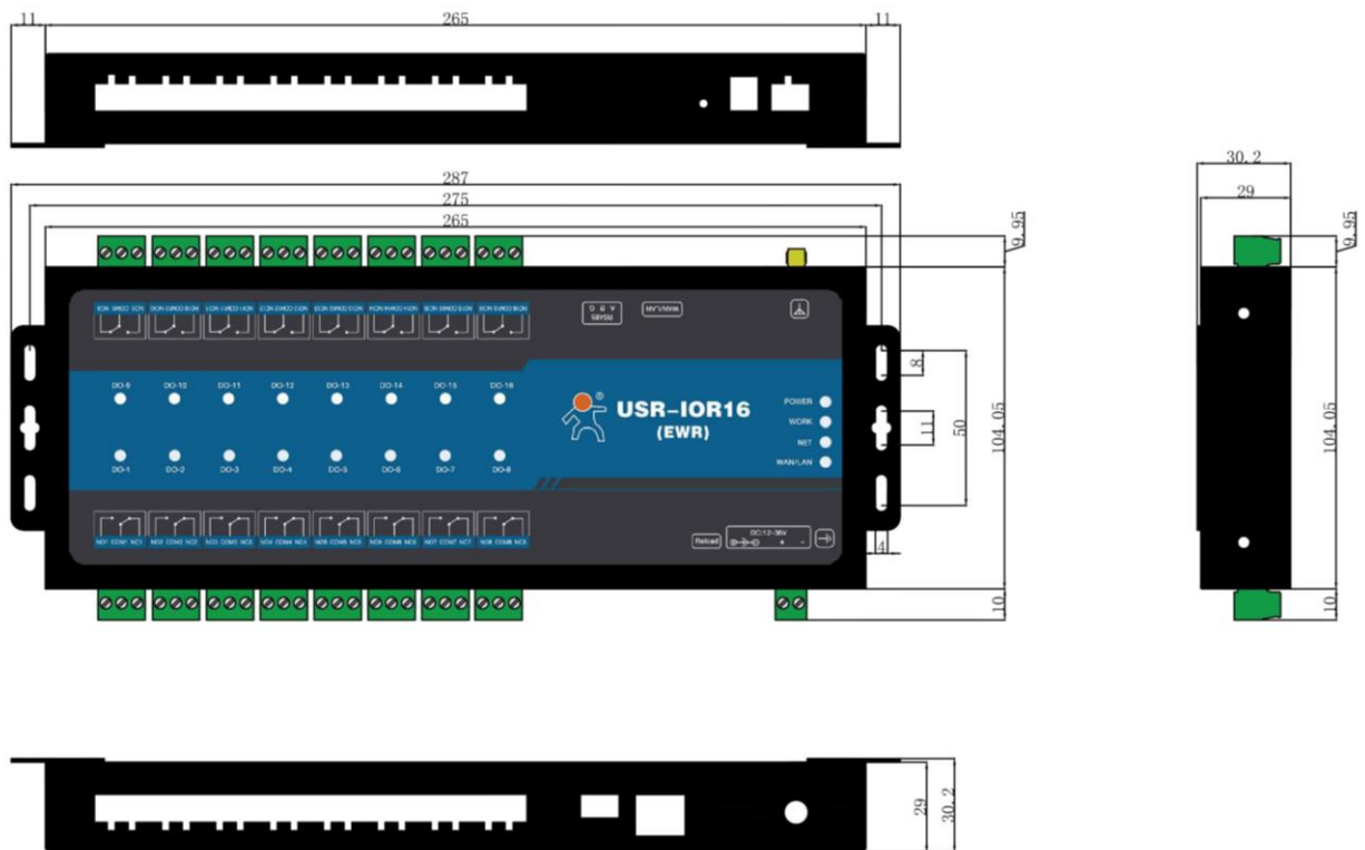
图 18 USR-IOR16-EWR 尺寸图
