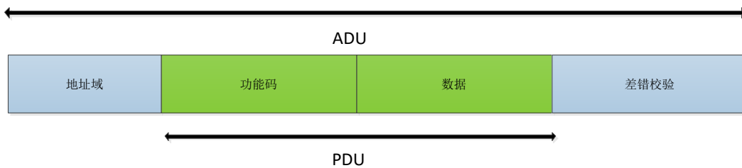
图 37 Modbus RTU 帧
