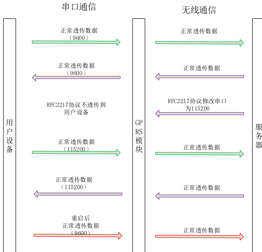
图 17 类 RFC2217 功能逻辑示意图
