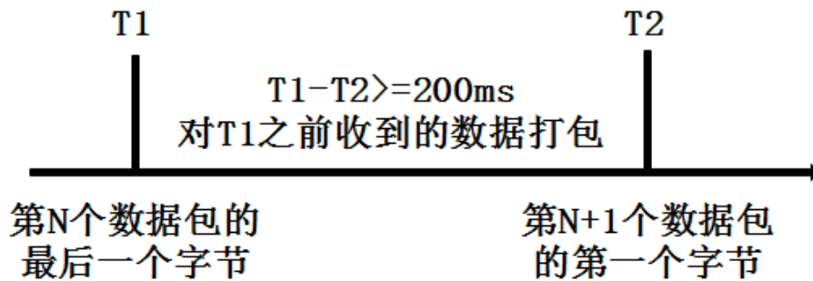
图 16 成帧机制示意图
