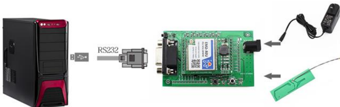
图 4 硬件连接示意图
