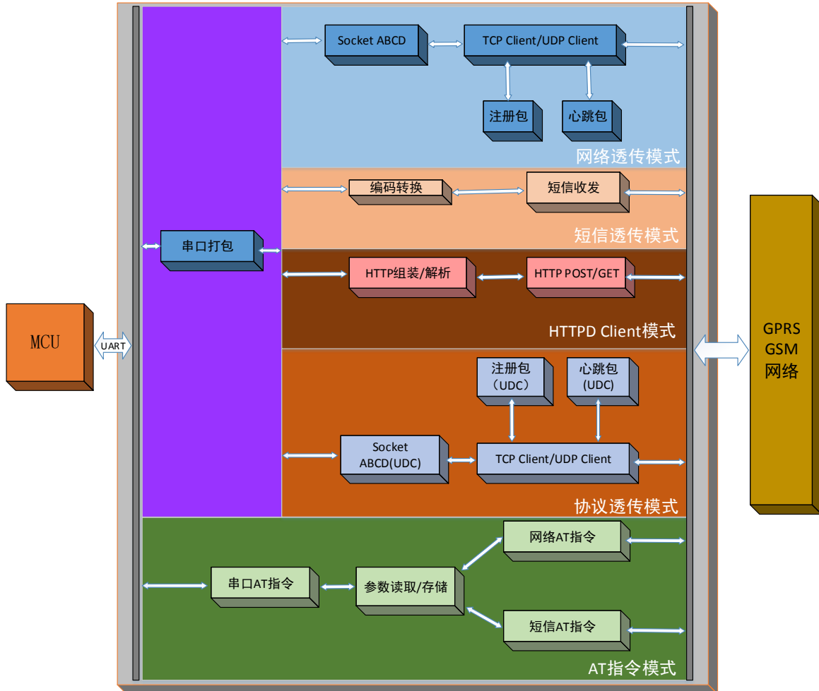
图 8 功能框图
