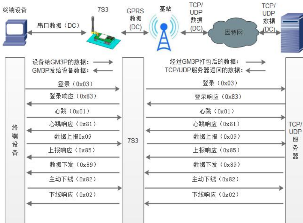
图 1 协议透传模式
