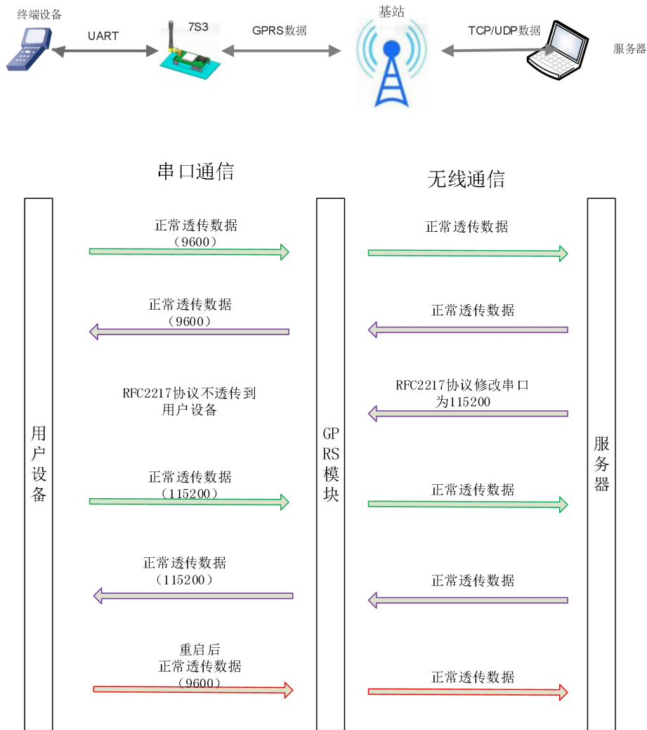
图 10 类 RFC2217 功能示意图
