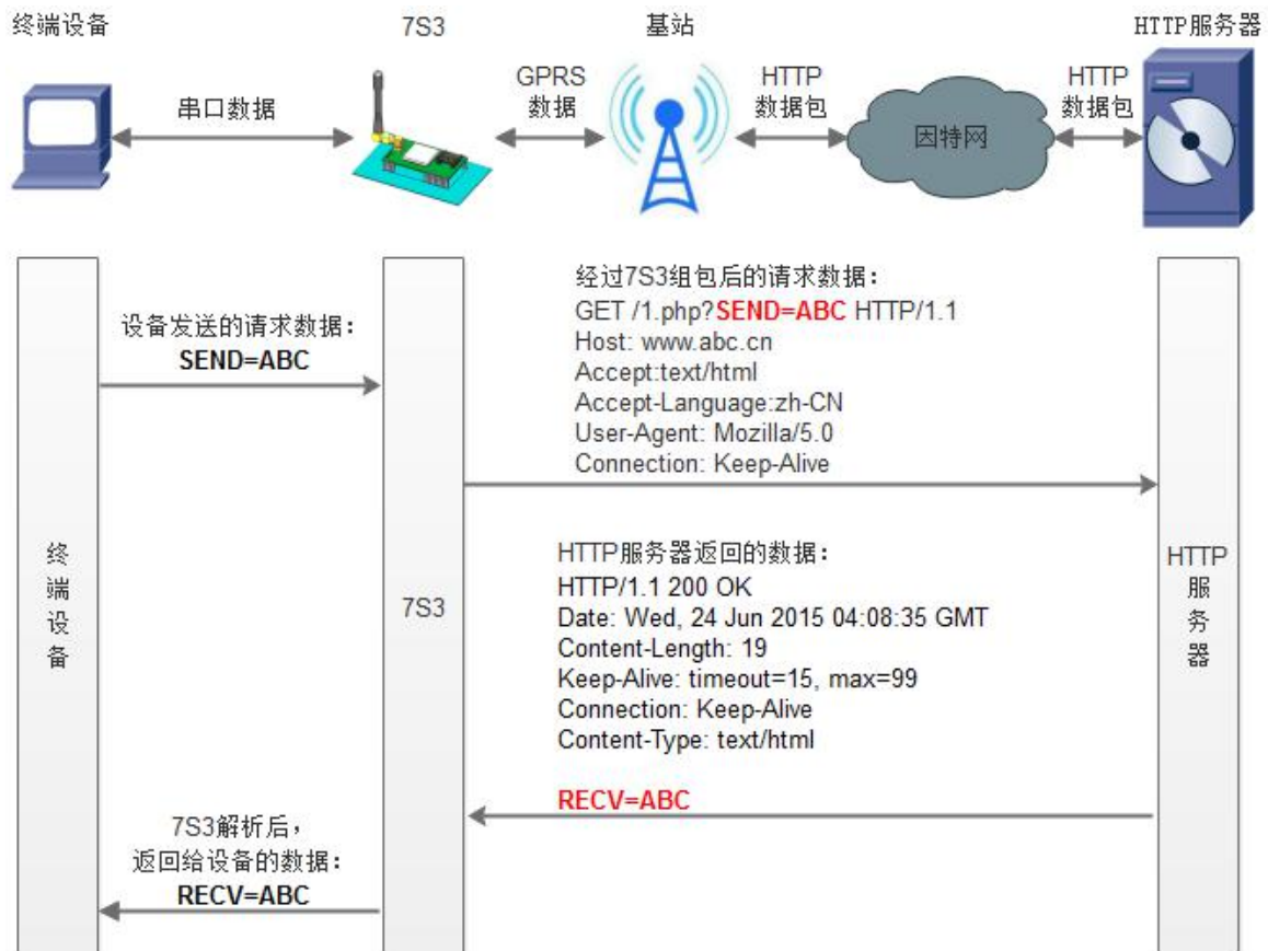
图 4 HTTPD 模式
