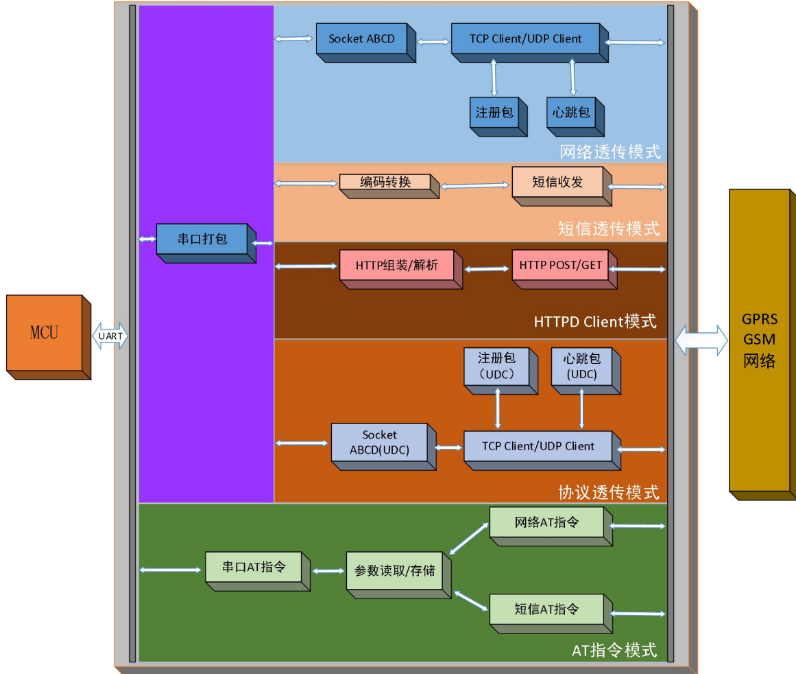
图 1 功能框图
