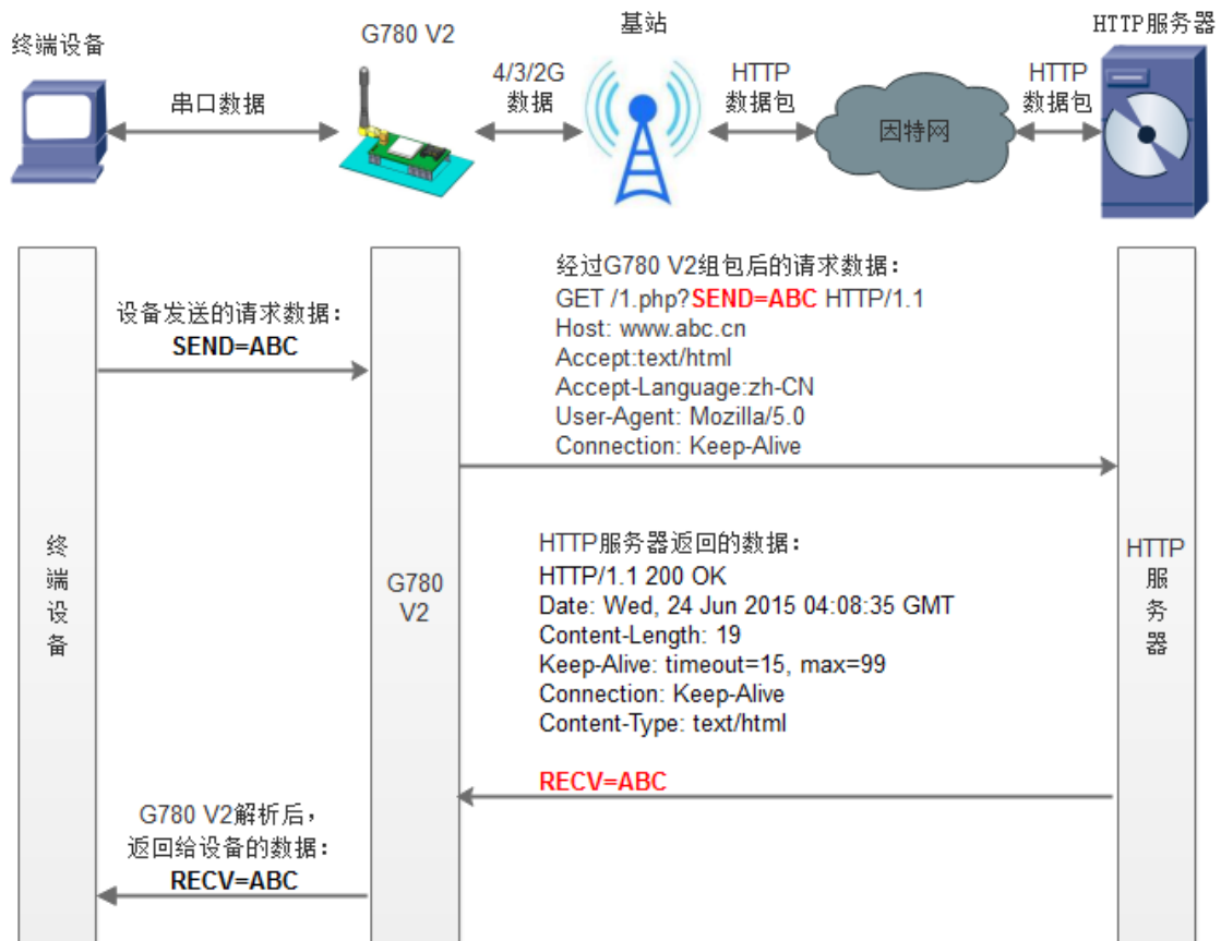
图 10 HTTPD 模式
