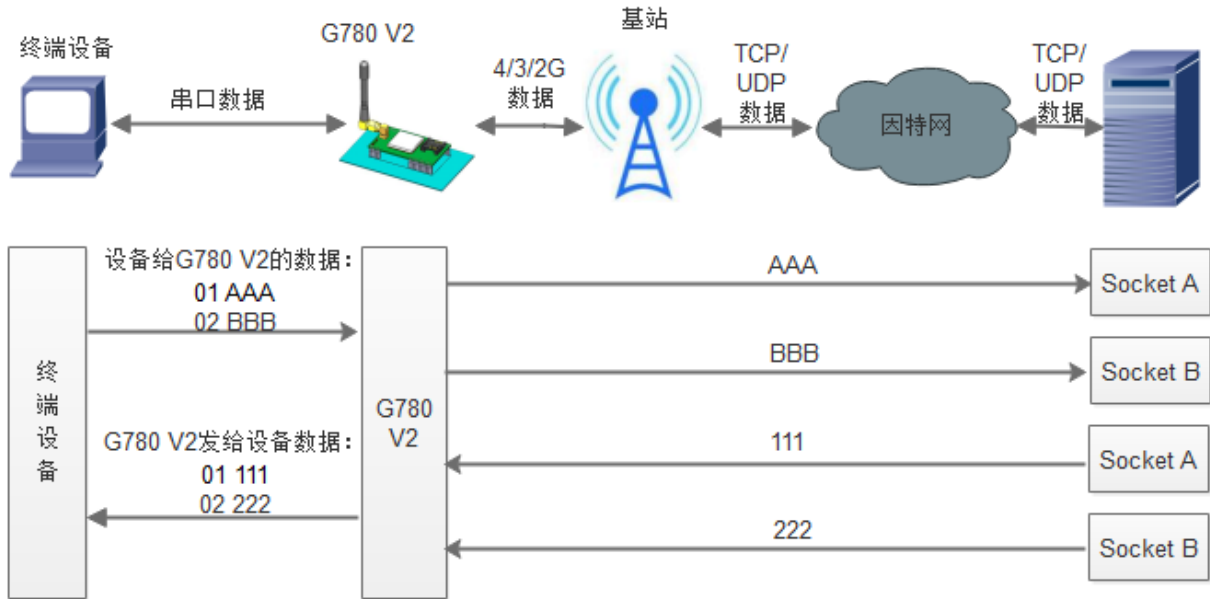
图 19 套接字分发协议示意图
