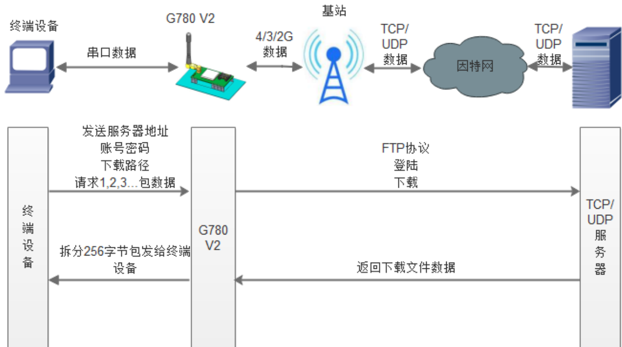
图 20 FTP 他升级协议示意图
