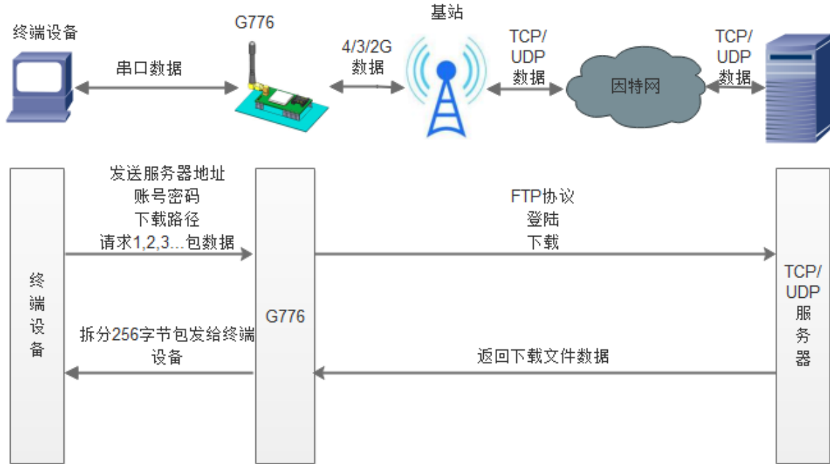
图 17 FTP 他升级协议示意图
