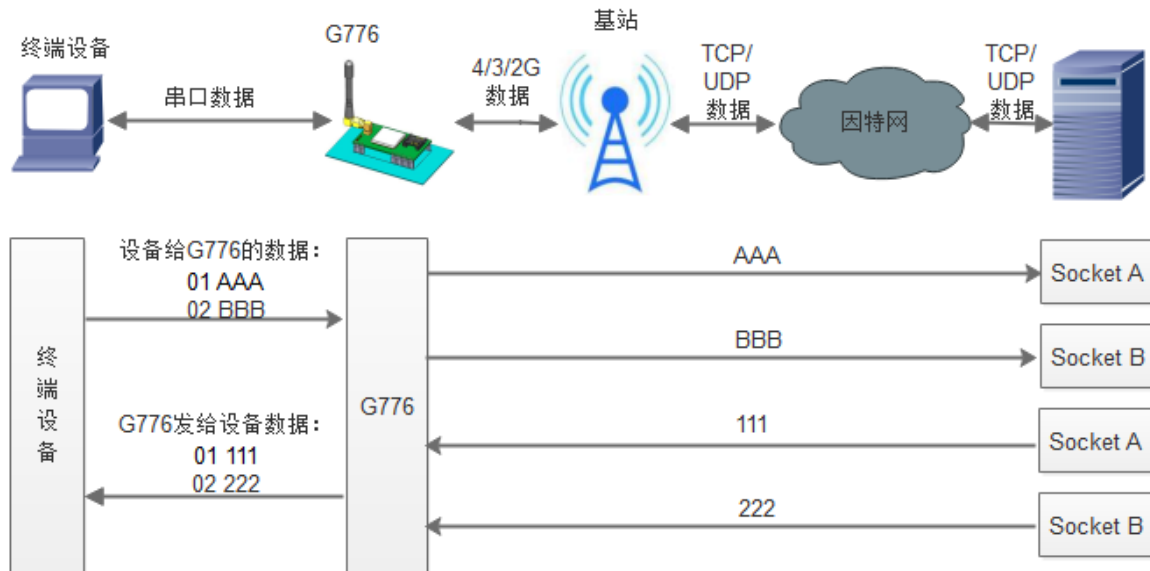
图 16 套接字分发协议示意图
