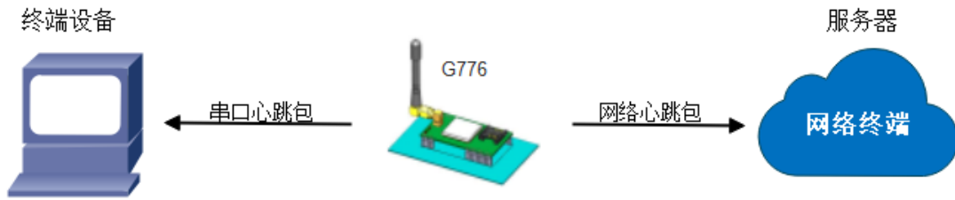
图 12 心跳包功能示意图
